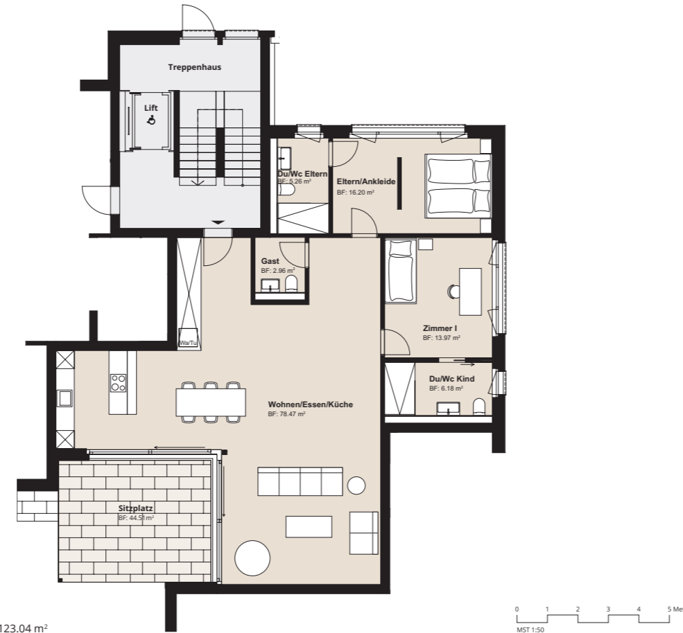
Wohnung 2 - Erdgeschoss Grundriss / Raumprogramm
