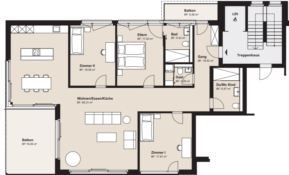
Wohnung 7 - 1. Obergeschoss Grundriss / Raumprogramm
