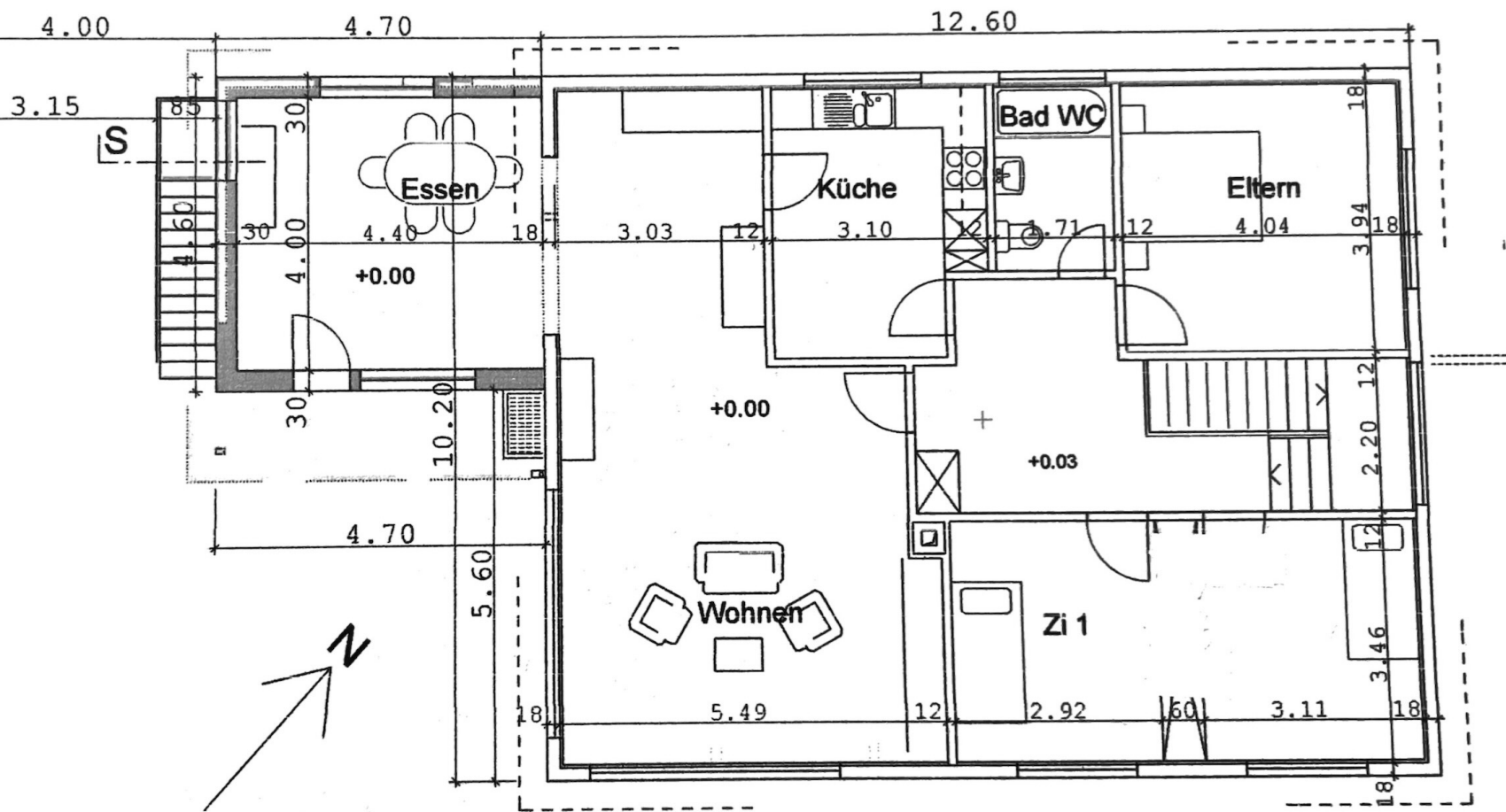
Grundriss EG
