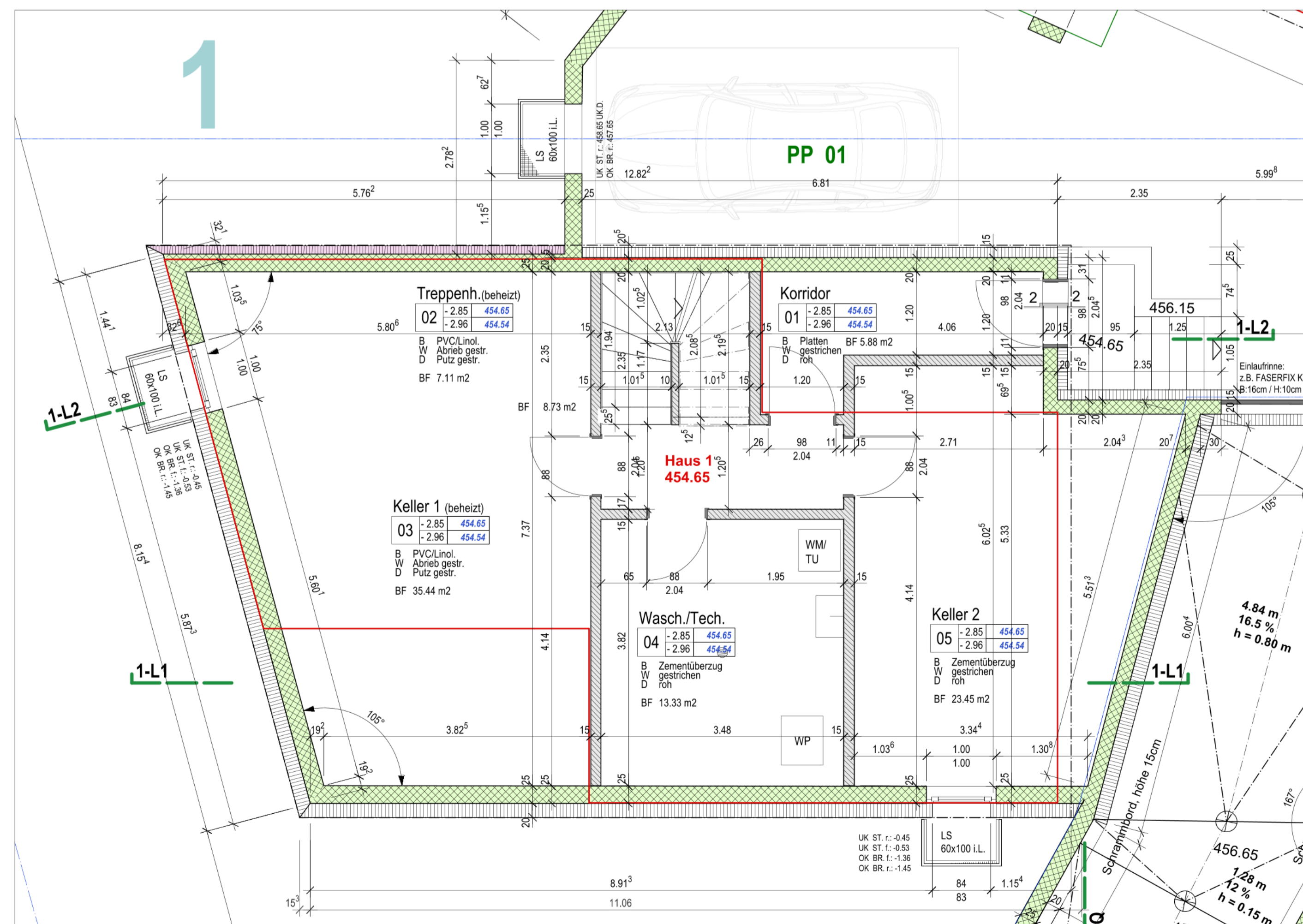
Untergeschoss
