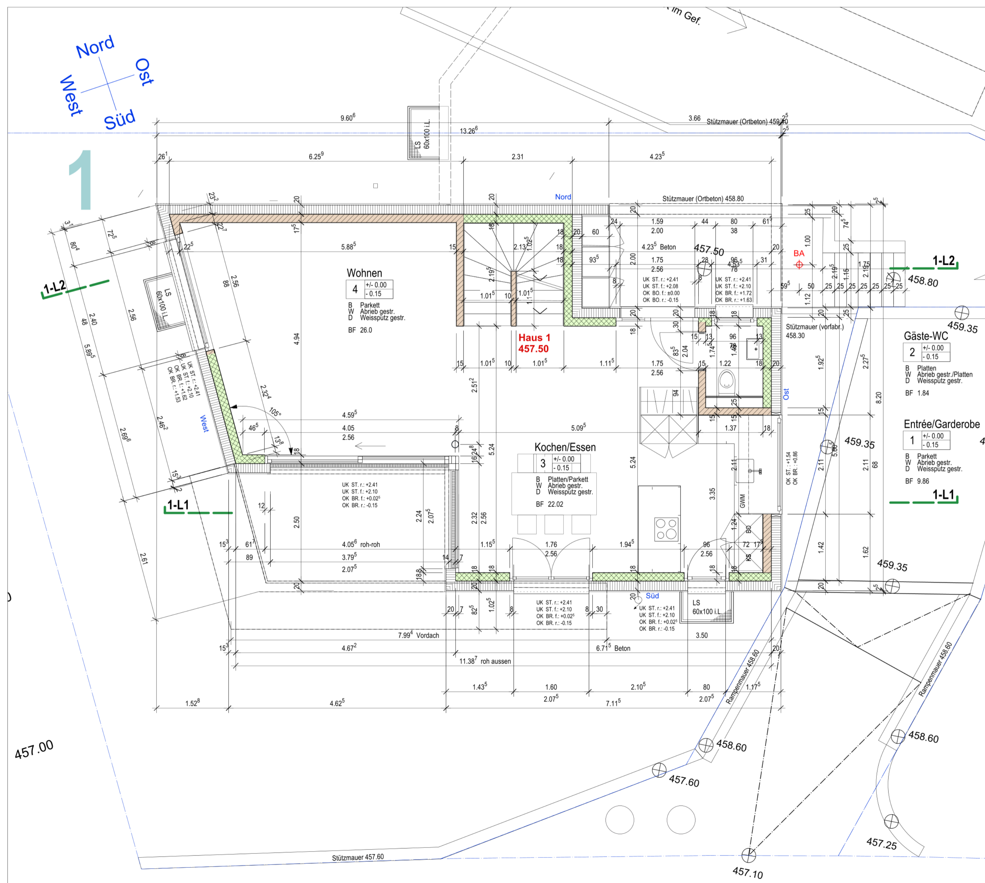
Erdgeschoss 1:50
