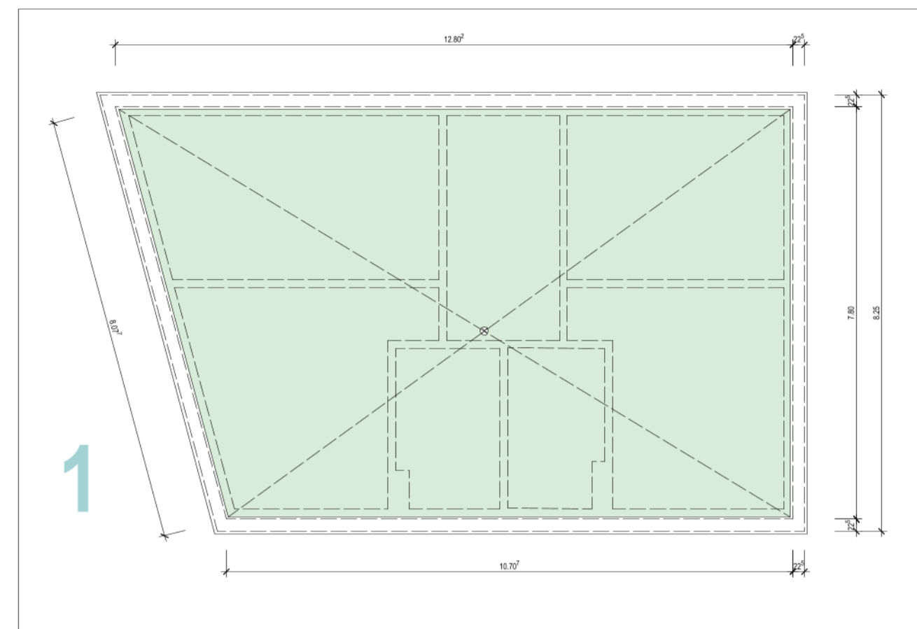
Dachaufsicht 1:100
