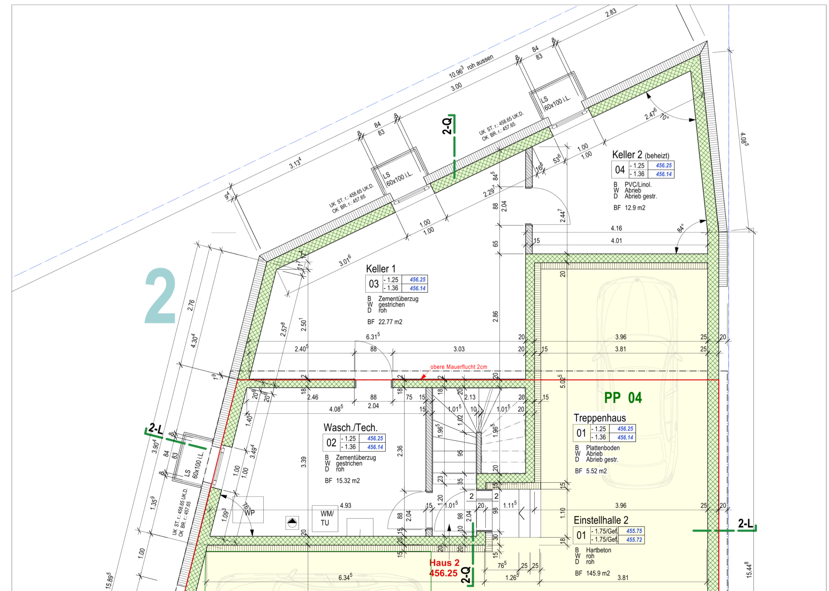
Untergeschoss
