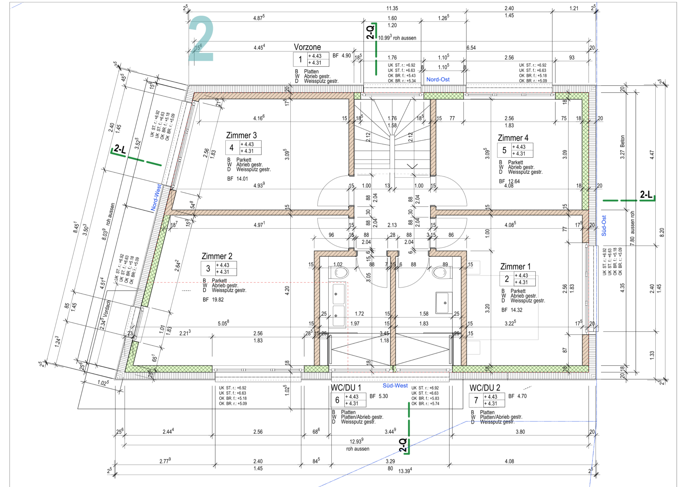
Obergeschoss
