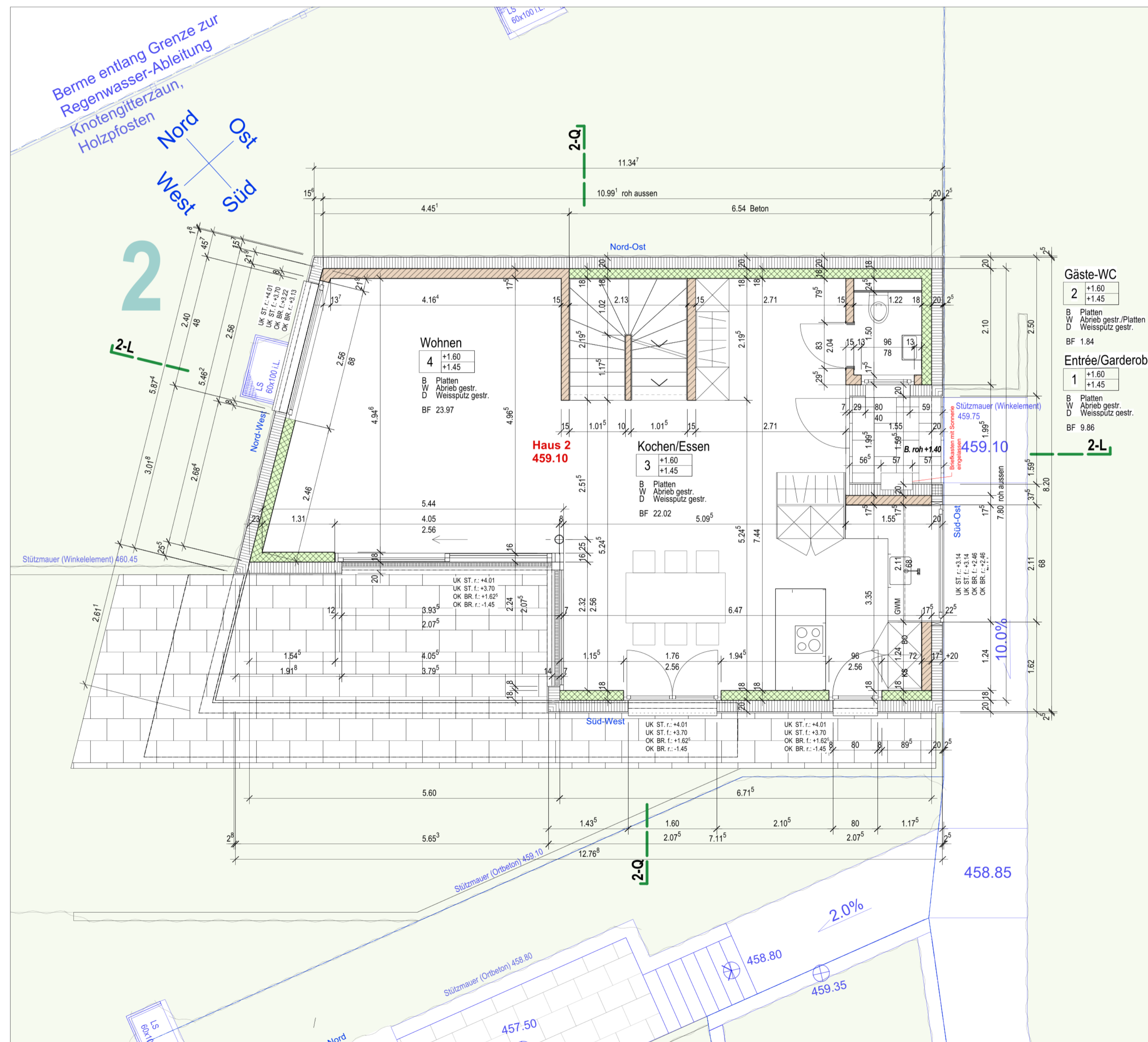
Erdgeschoss 1:50
