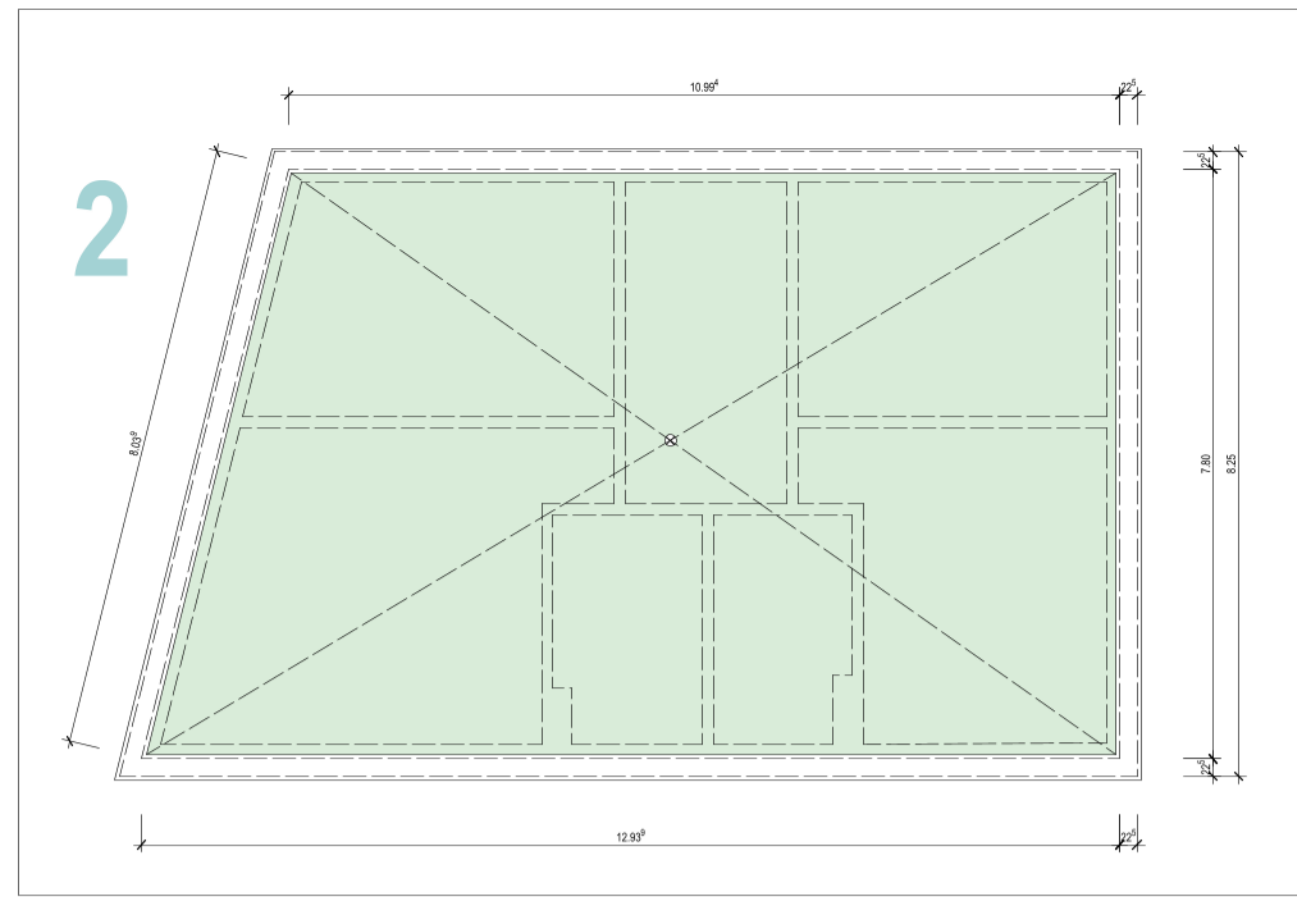
Dachaufsicht 1:100
