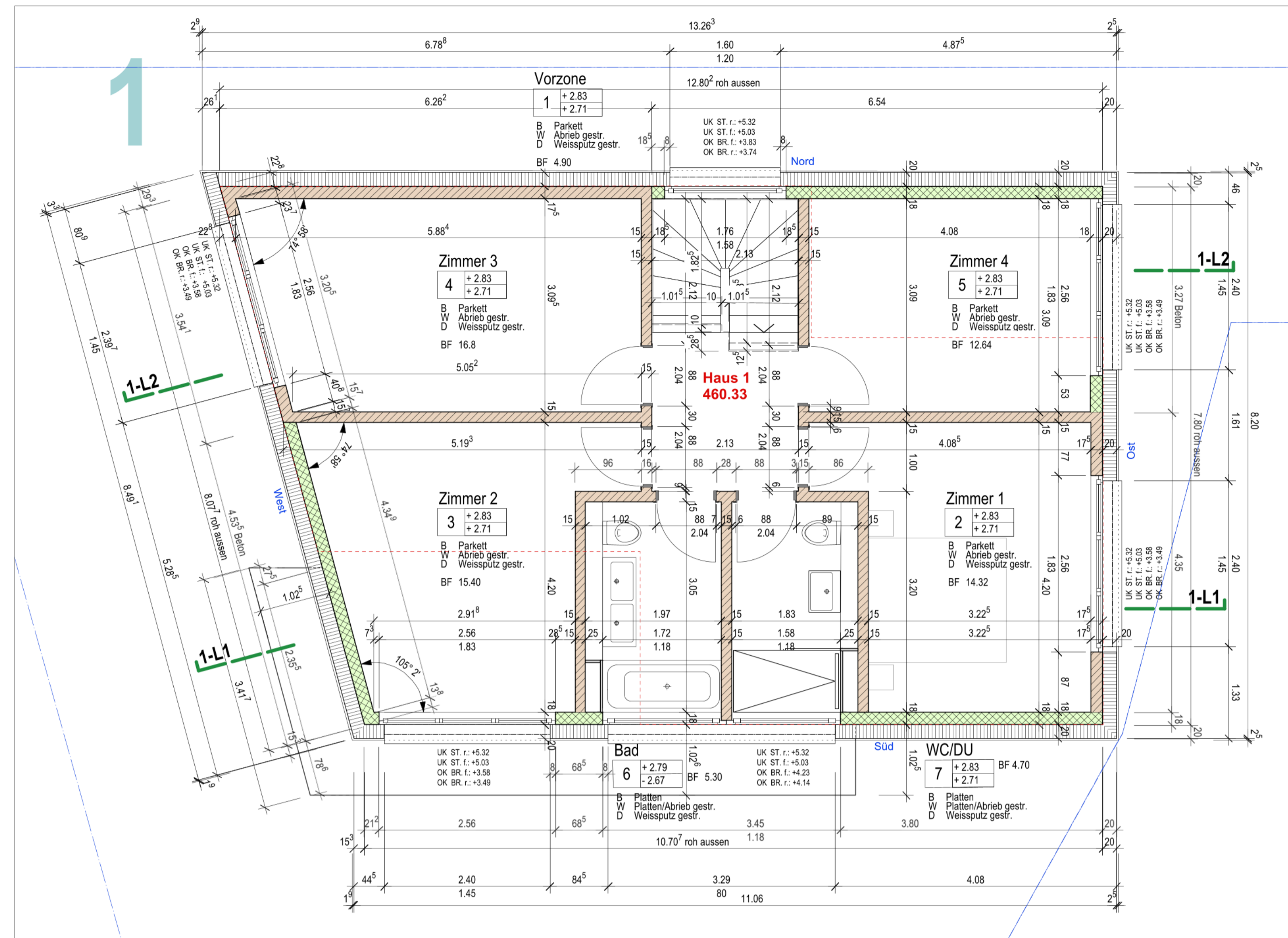
Obergeschoss
