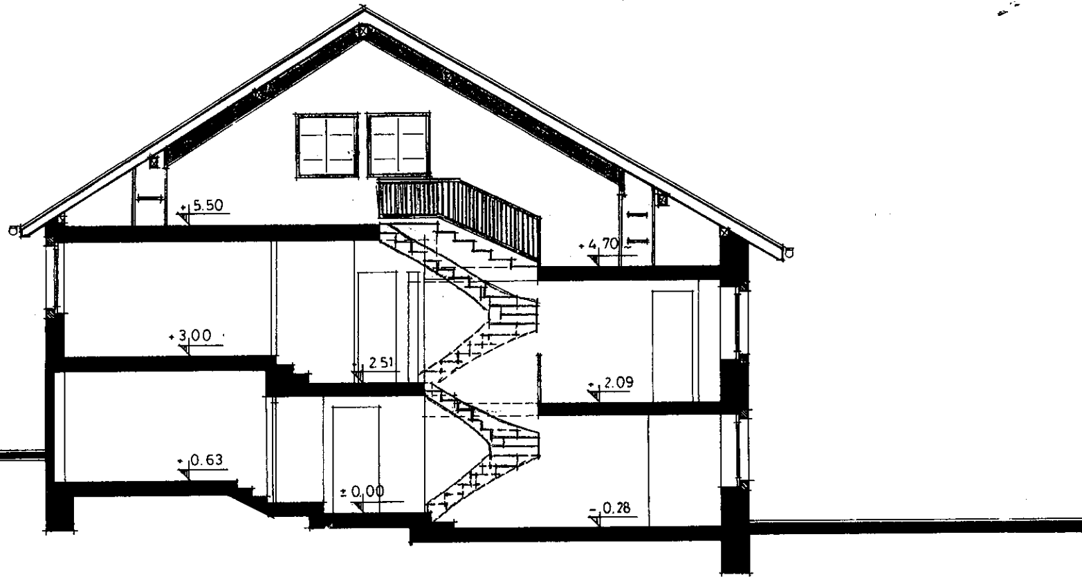
COUPE CC
