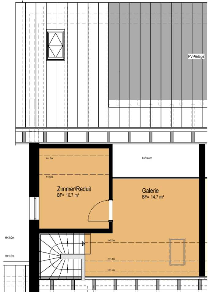
2.Dachgeschoss 25.4 m²
