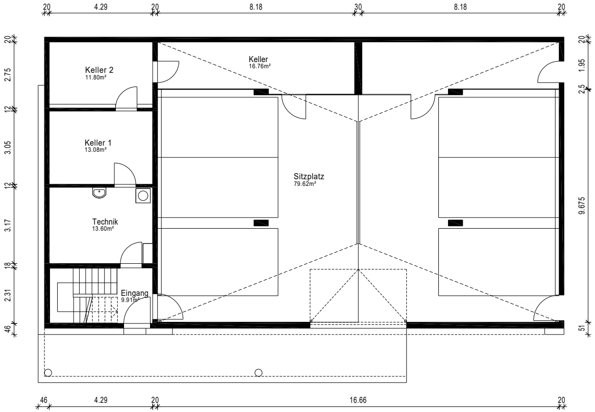
Kellergeschoss
