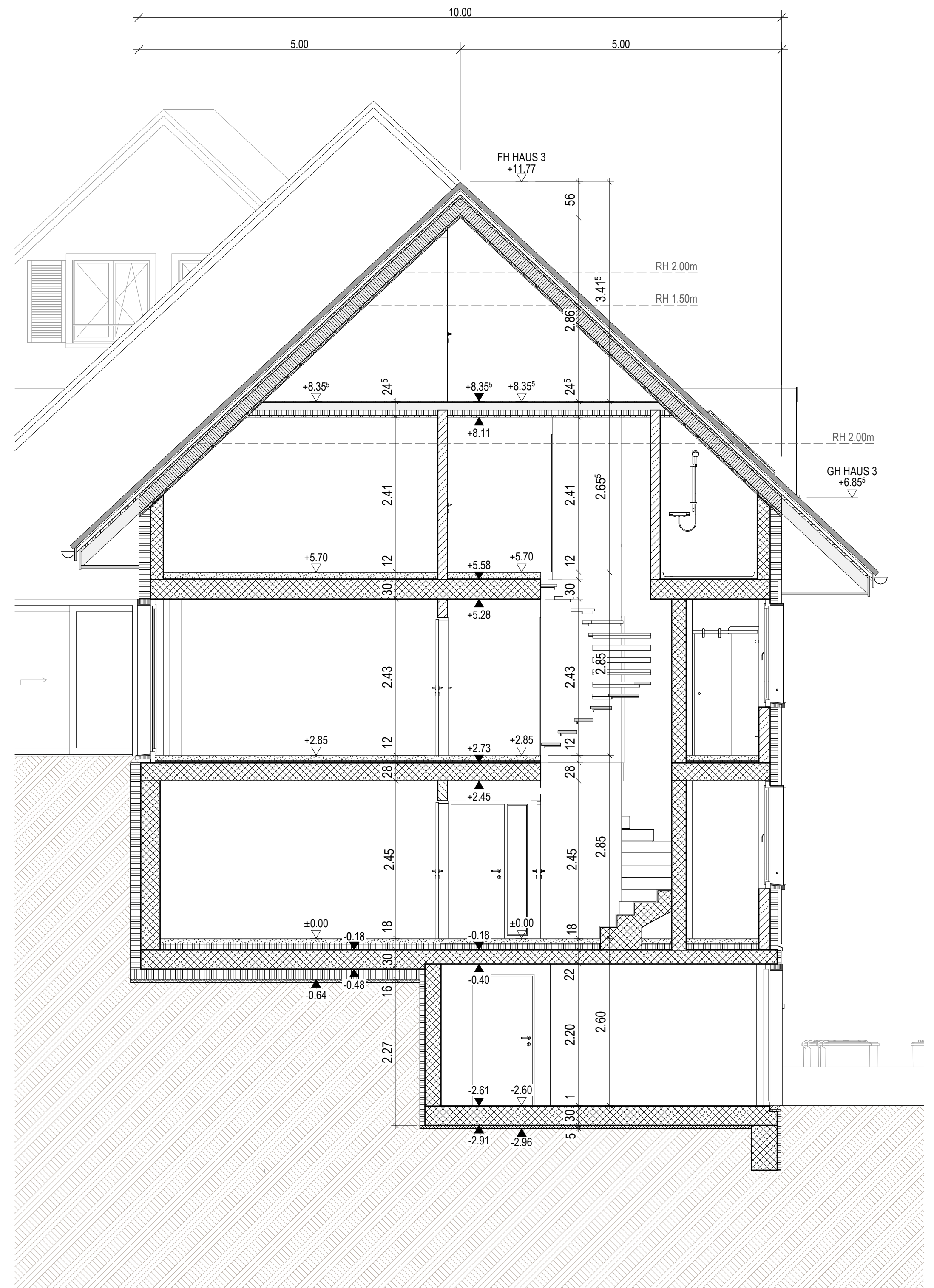
D HAUS 3 SCHNITT D - D
