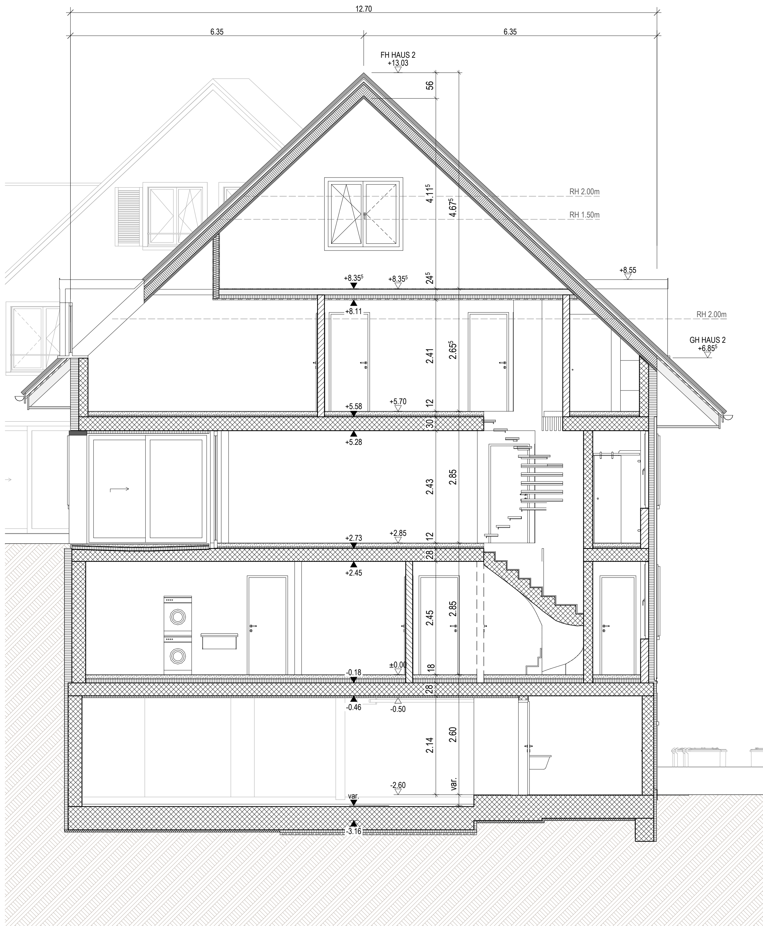
C HAUS 2 SCHNITT C - C
