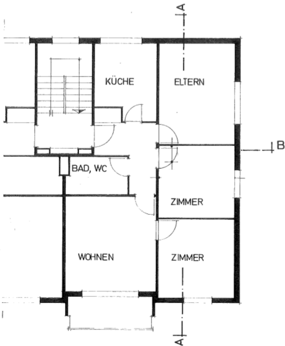
WOHNUNGSGRUNDRISS 2.OBERGESCHOSS
