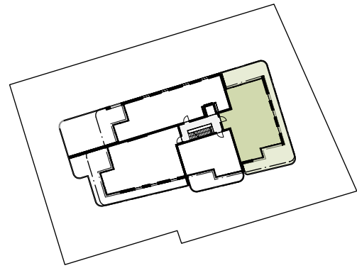
ÜBERSICHTSPLAN OG1 1:1000
