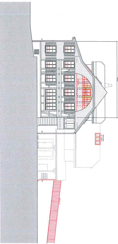
fassade süd
