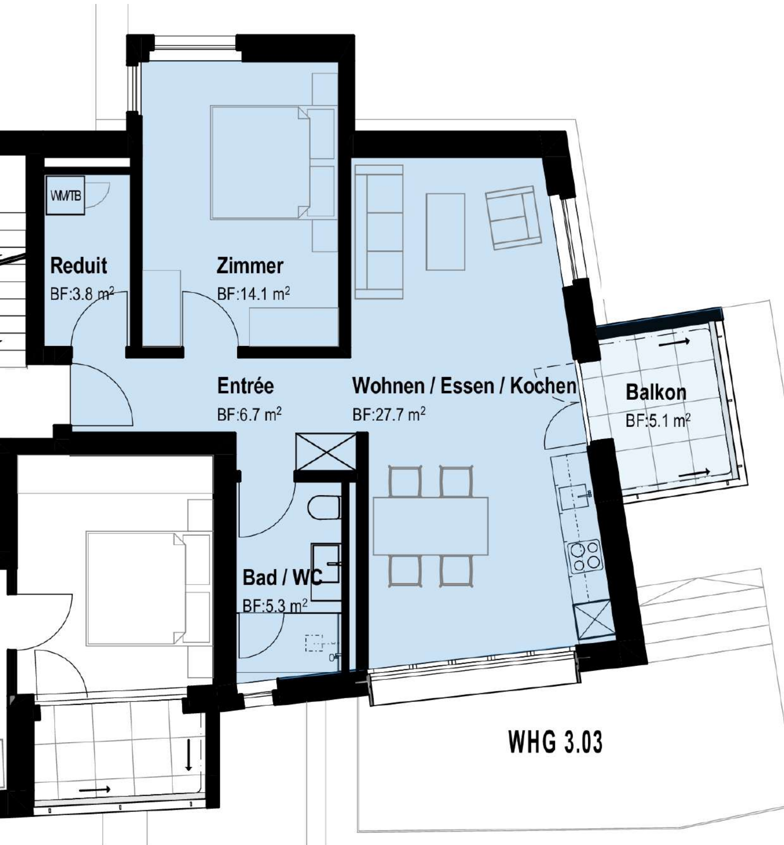
Rosengartenstrasse 55, Zürich Grundriss 3.Obergeschoss
