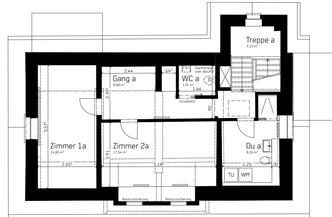
Dachgeschoss
