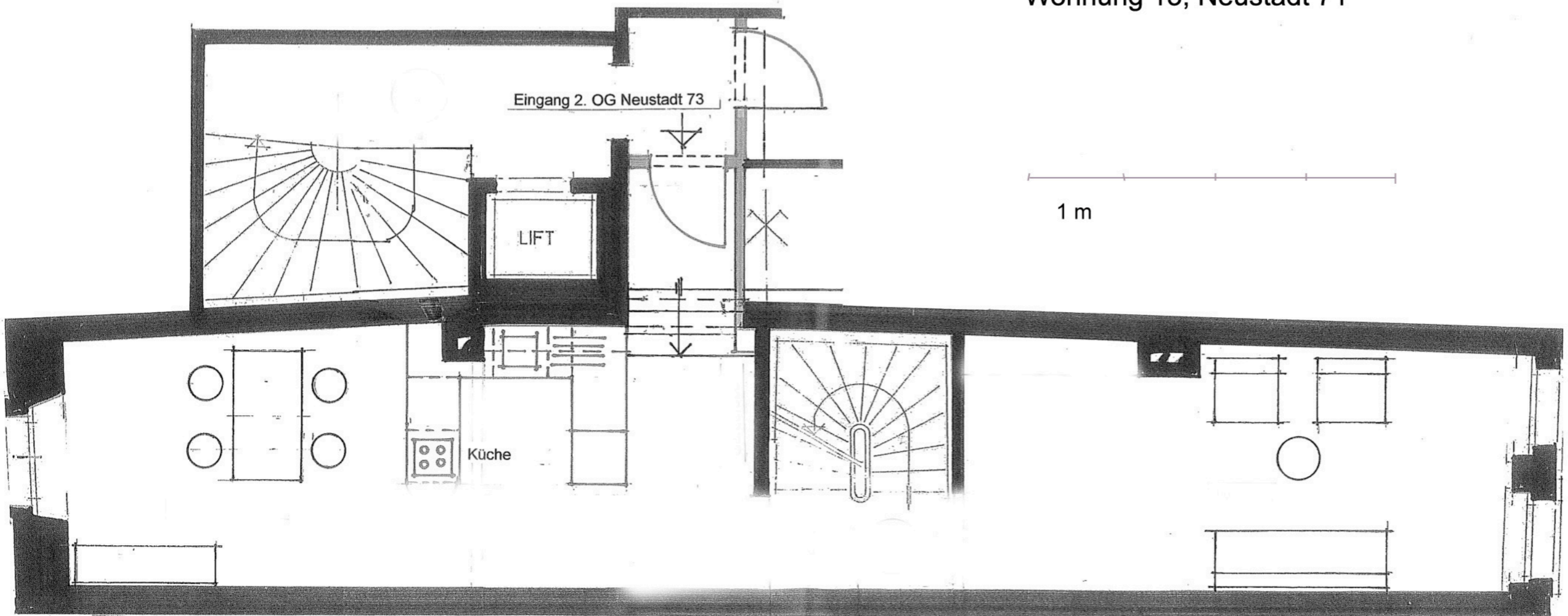
Grundriss 2. Obergeschoss
