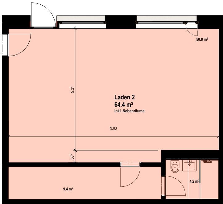
Grundriss M. 1:100
