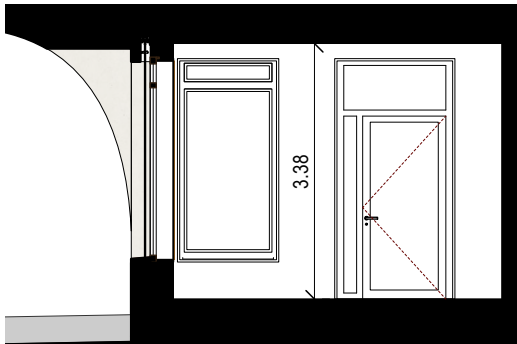
Schnitt M. 1:100
