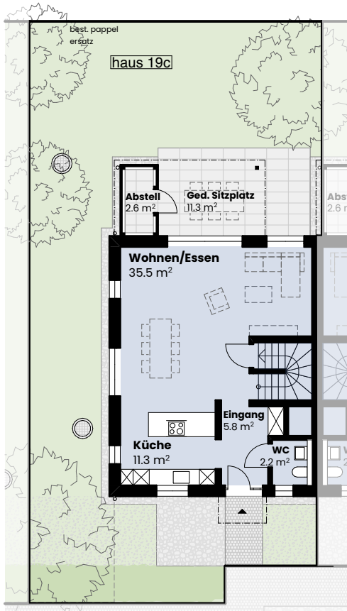
Erdgeschoss
