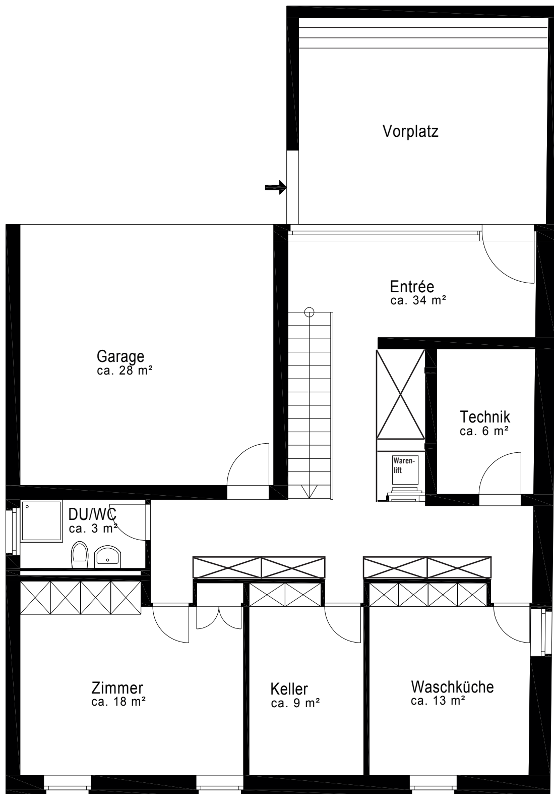
Erdgeschoss Doppel-Einfamilienhaus, Männedorf nicht massstäblich
