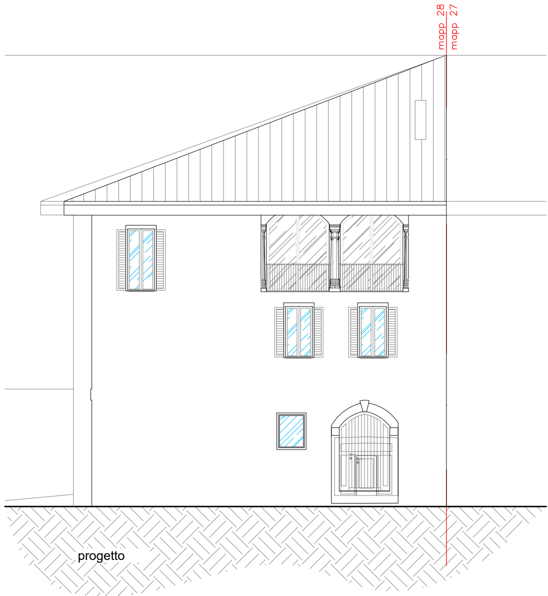
PROSPETTO NORD-EST
