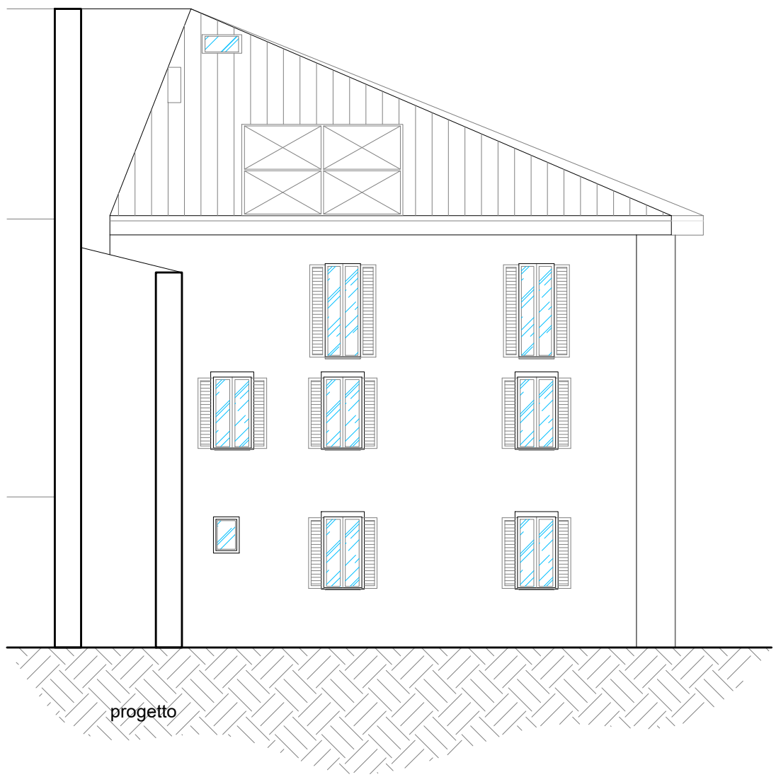
PROSPETTO SUD-EST
