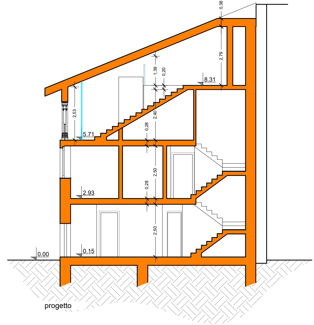
SEZIONE
