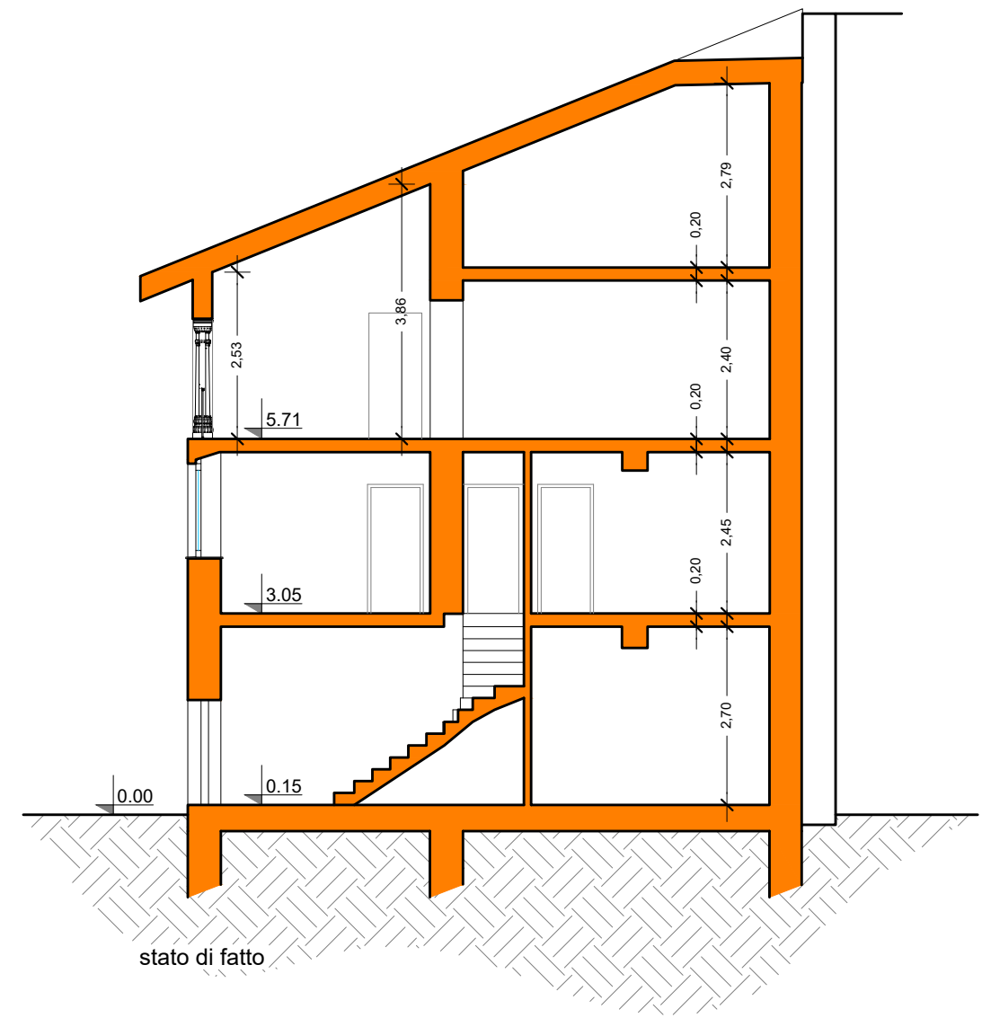
SEZIONE
