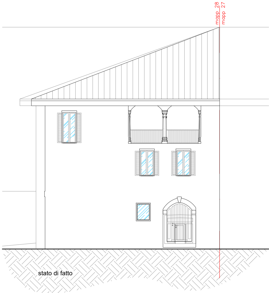
PROSPETTO NORD-EST
