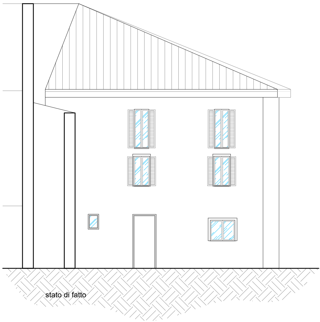
PROSPETTO SUD-EST
