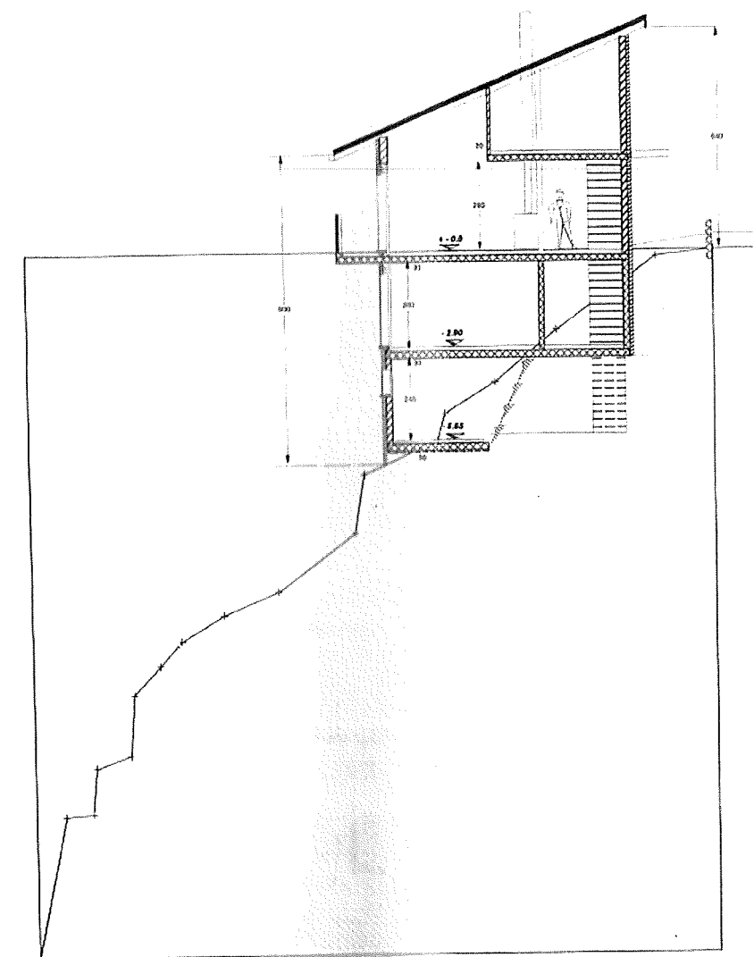
casa monofamiliare mapp. 430 M.to Carasso sezione trasversale A-A 1:100 11.01.03
