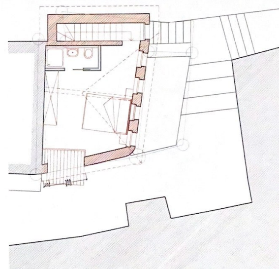
SECONDO PIANO
