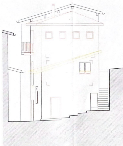
FACCIATA EST
