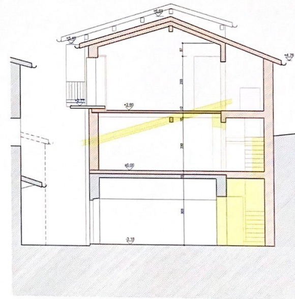
SEZIONE
