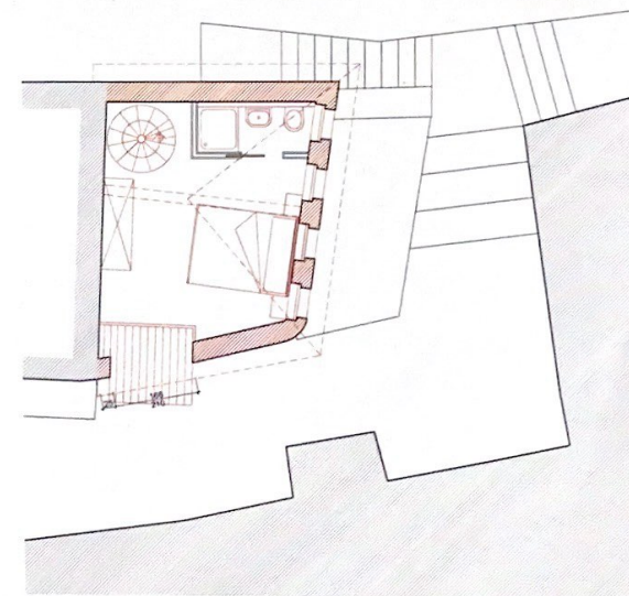
SECONDO PIANO
