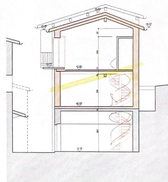
SEZIONE
