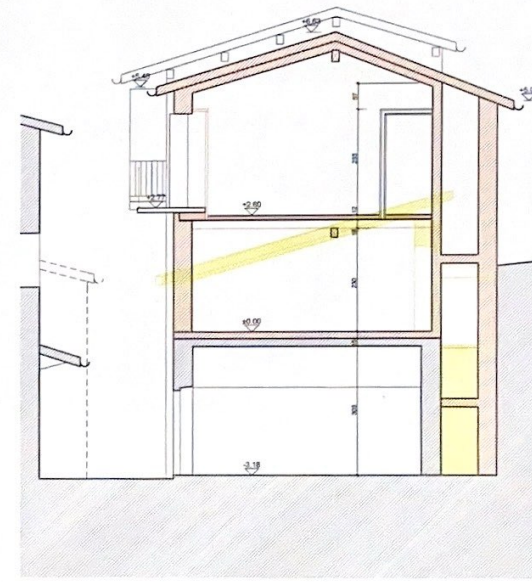
SEZIONE
