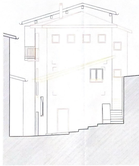
FACCIATA EST
