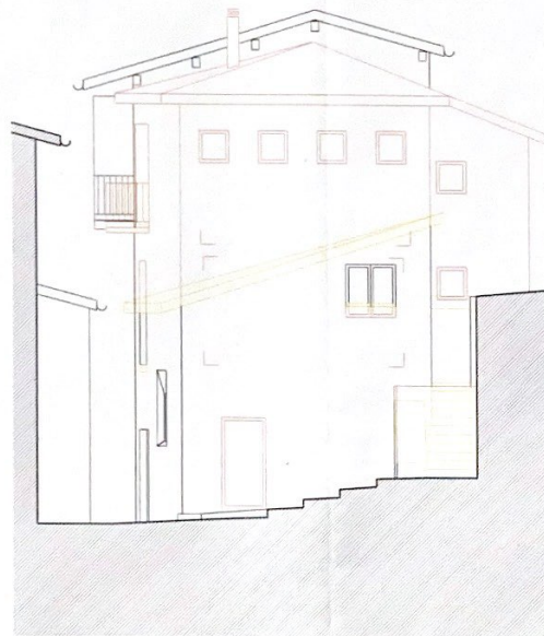
FACCIATA EST
