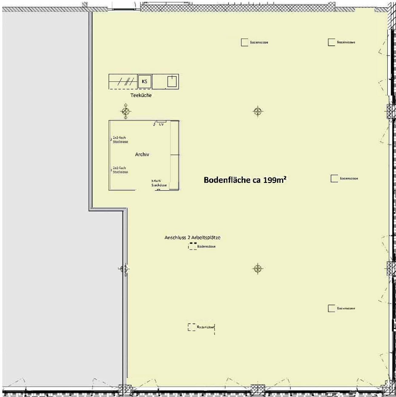
Grundriss Büro
