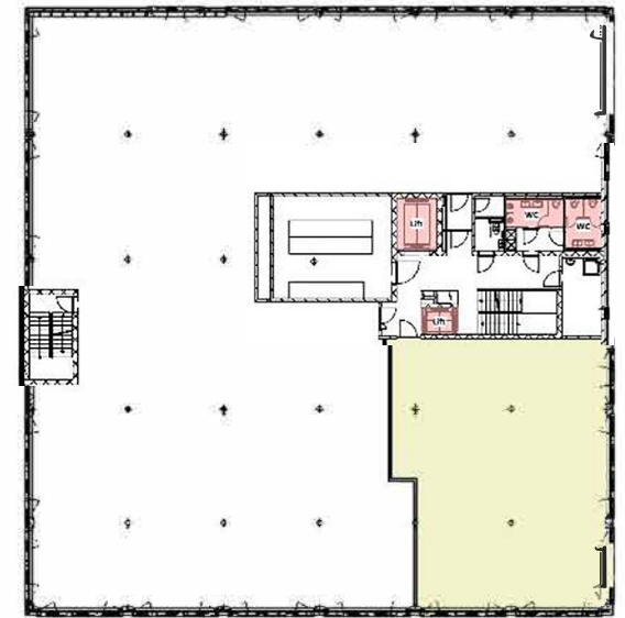
Situation 2. Obergeschoss
