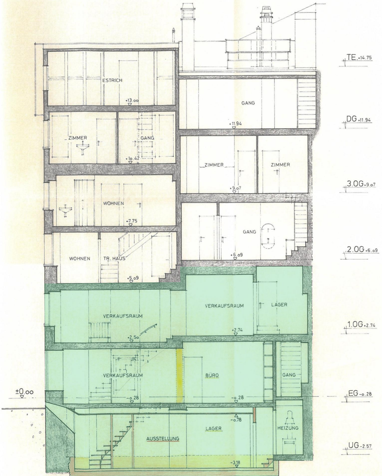
SCHNITT A-A
