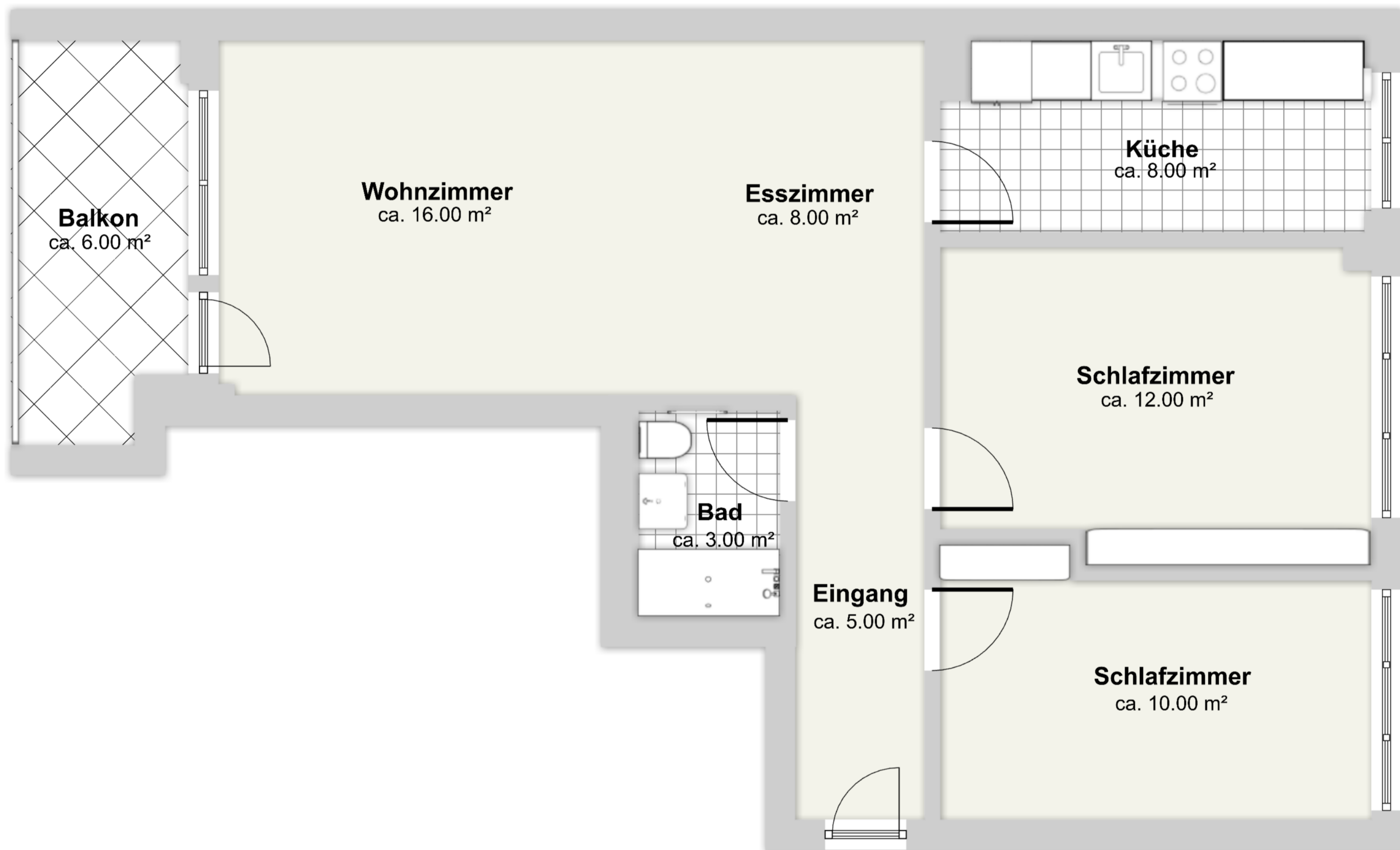
1. Obergeschoss
