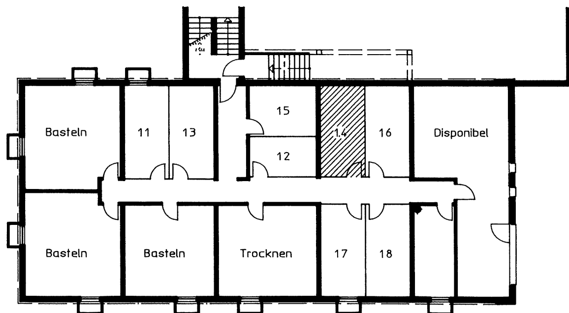
Keller Haus 1
