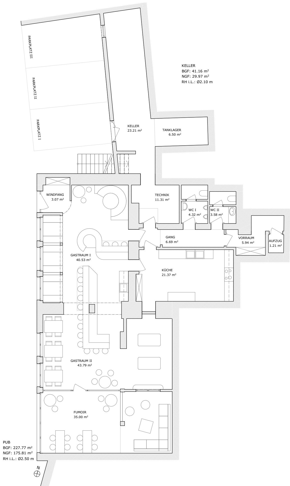
VIKTORIA GRUNDRISS PUB 0.EG MASSSTAB 1:125 | FORMAT A4 | DATUM 25.03.2024
