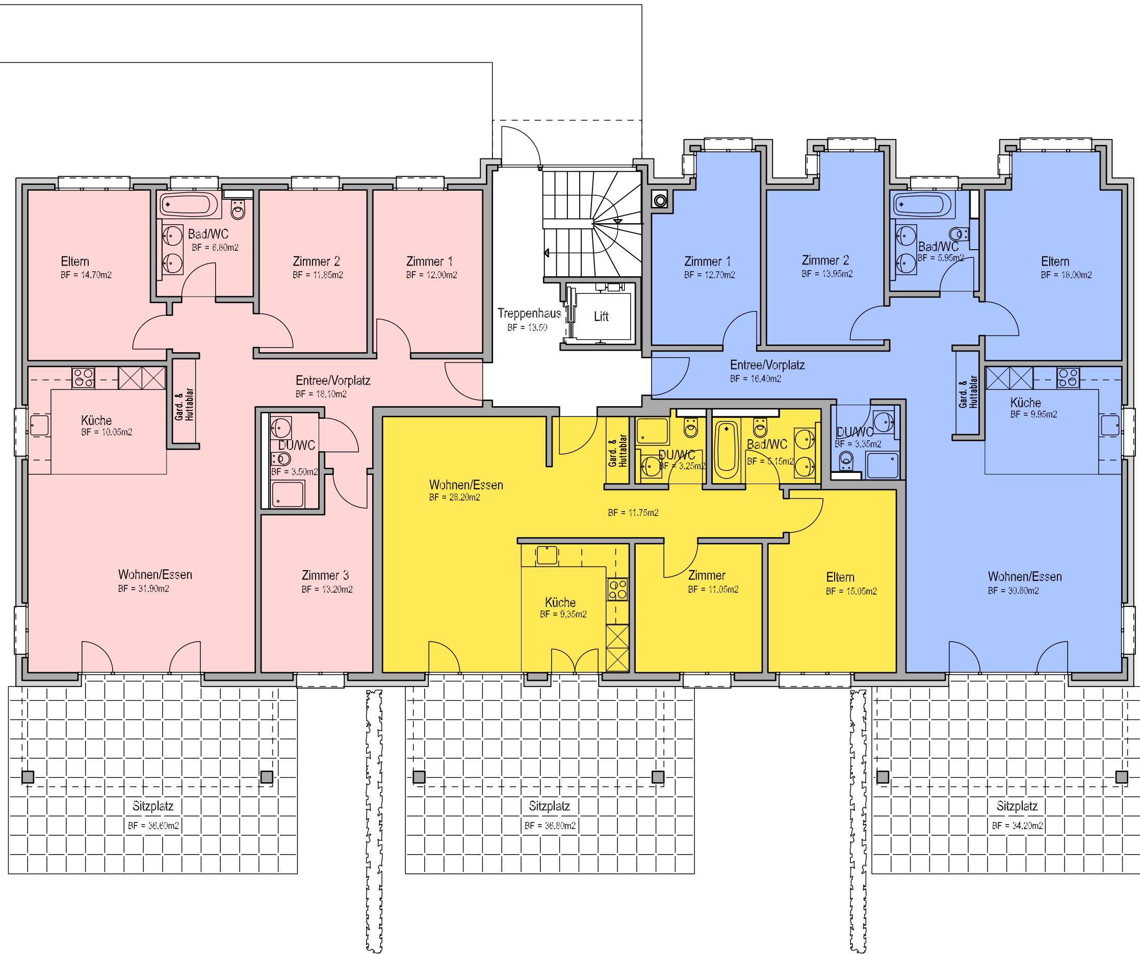
ERDGESCHOSS / HAUS 3 / 1 : 100
