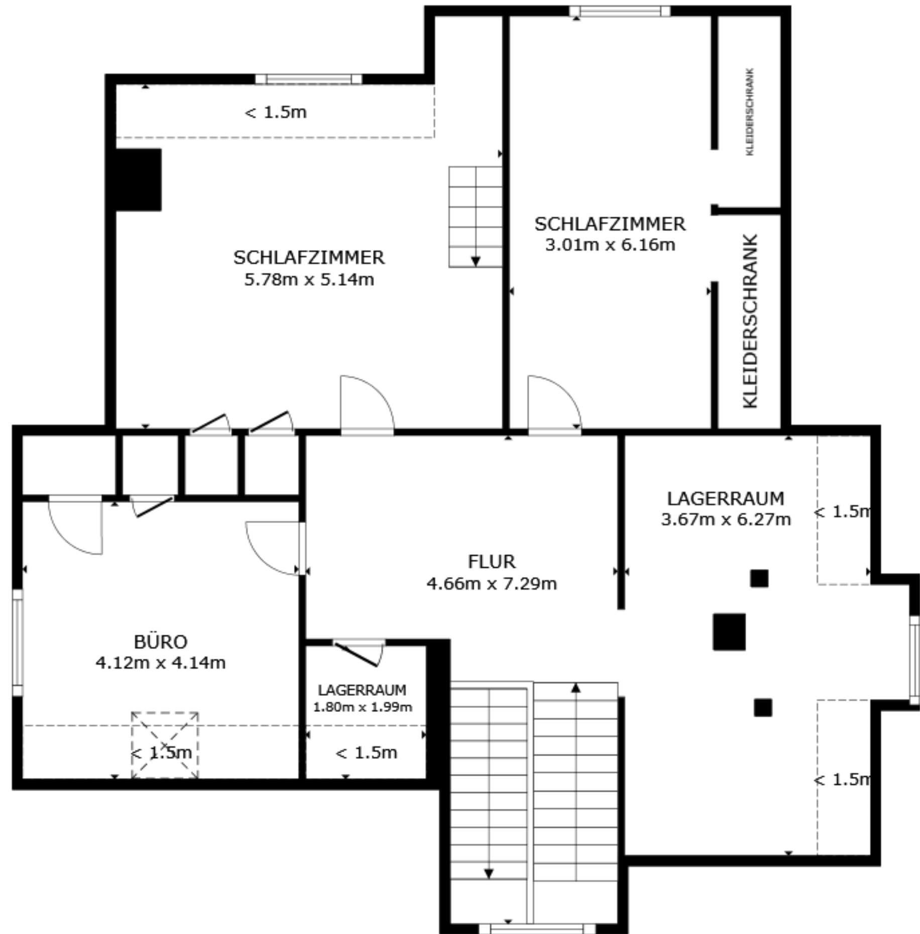
STOCKWERK 4
