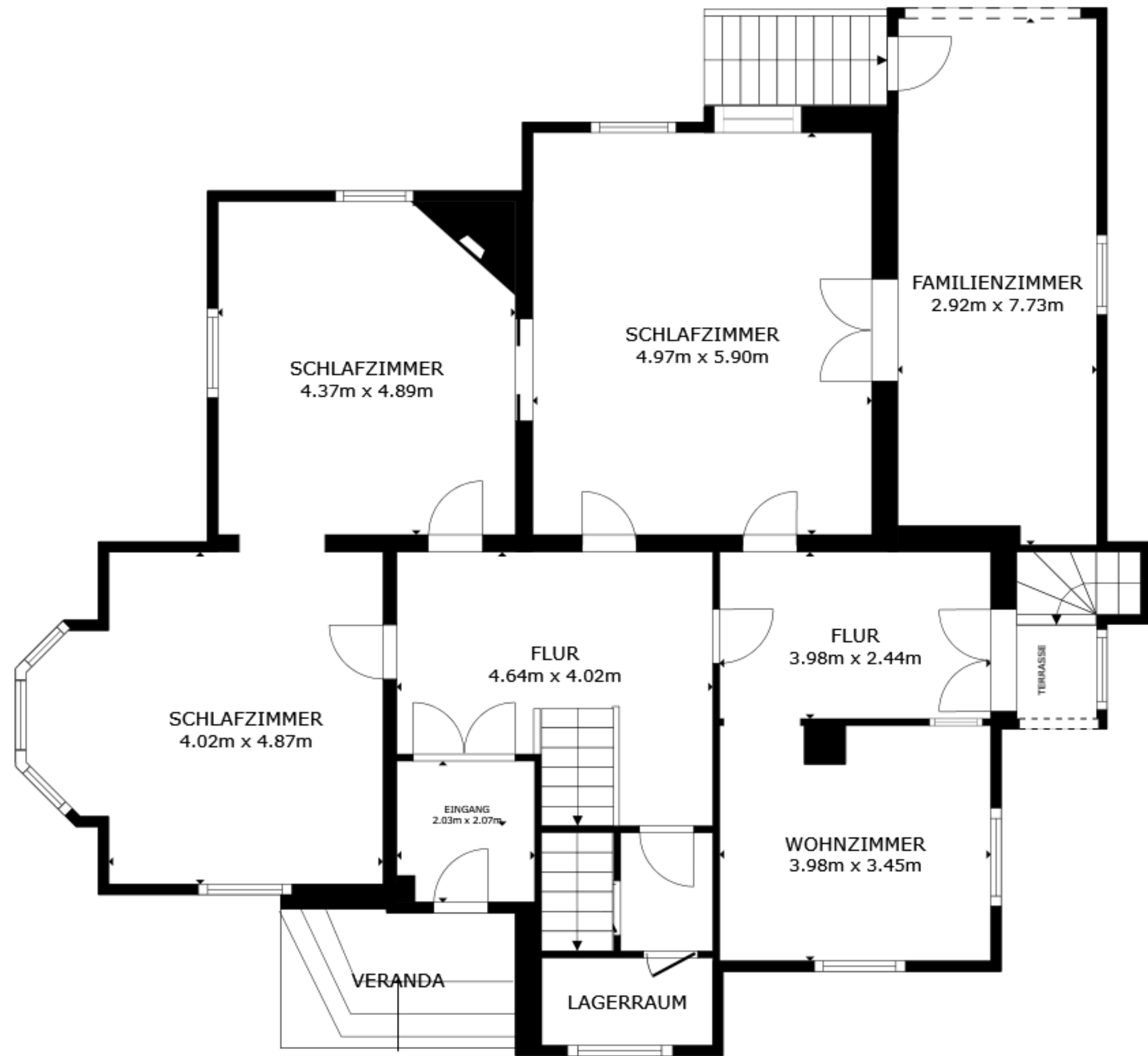
STOCKWERK 2
