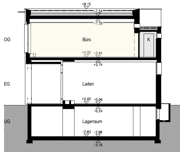
Schnitt C-C
