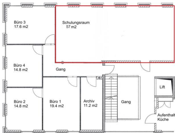
Grundriss 1. Obergeschoss, Büro mit 57 m 2
