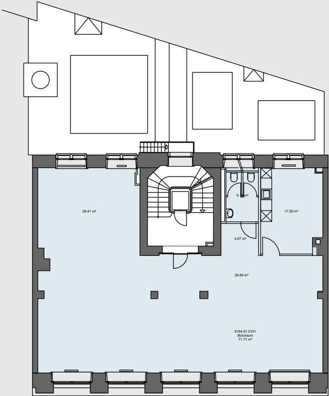
1. Obergeschoss
