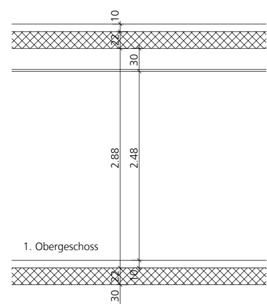
Prinzipsschnitt 1:50
