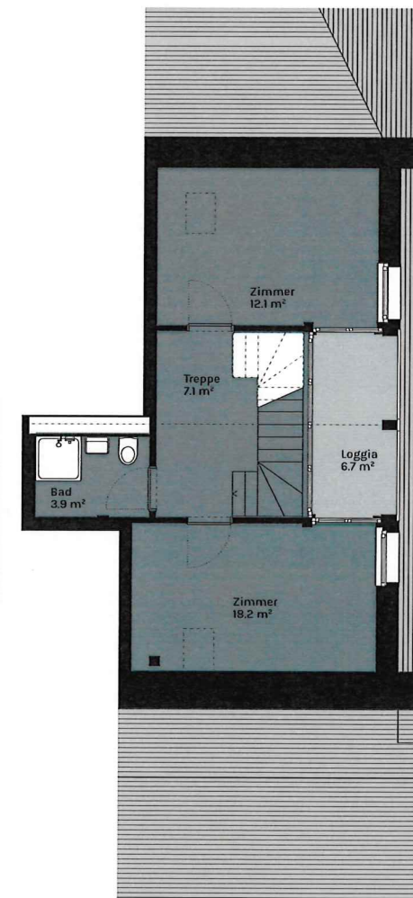
2. Obergeschoss
