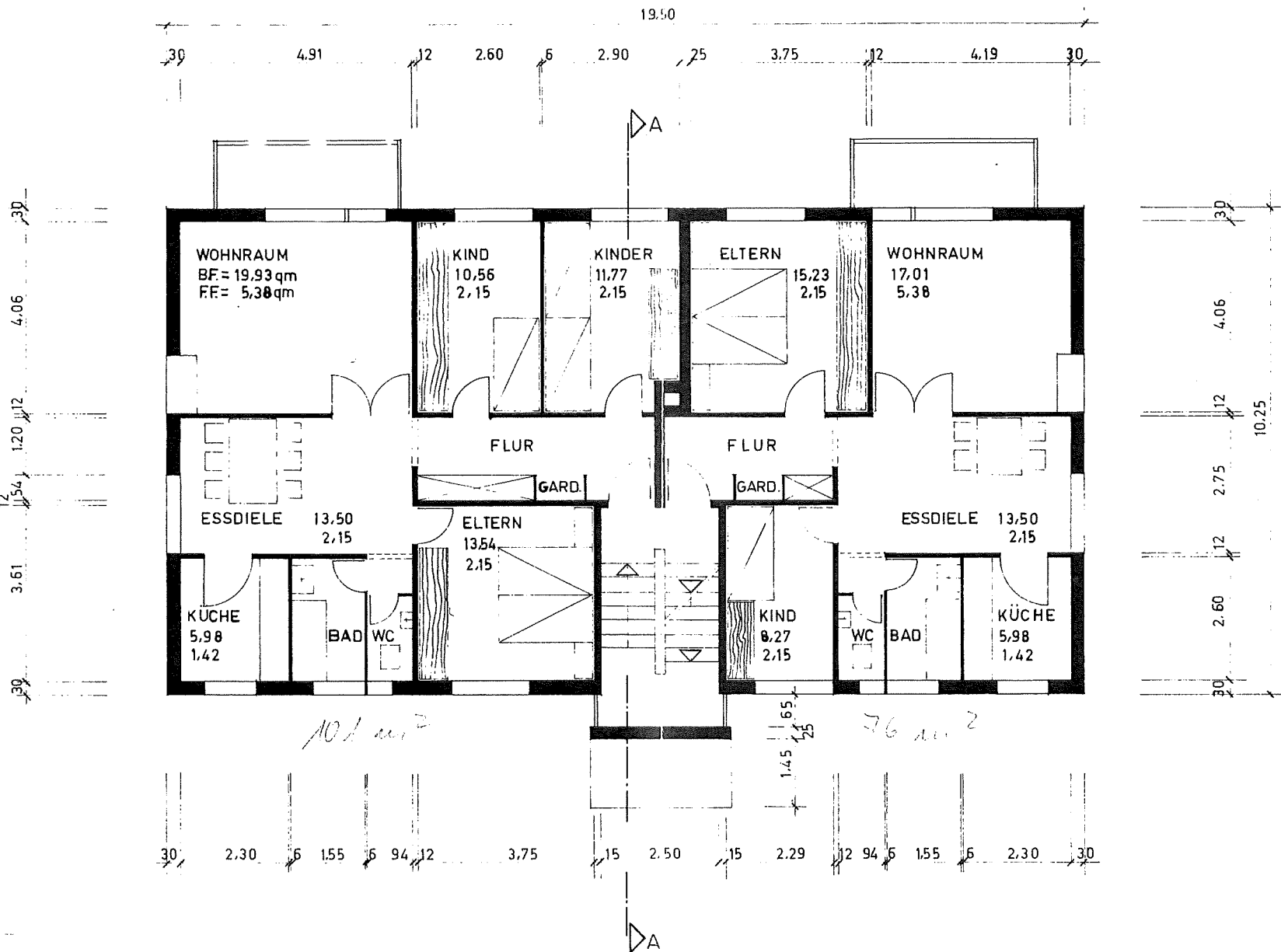
ERDGESCHOSS, 1. UND 2. OBERGESCHOSS
