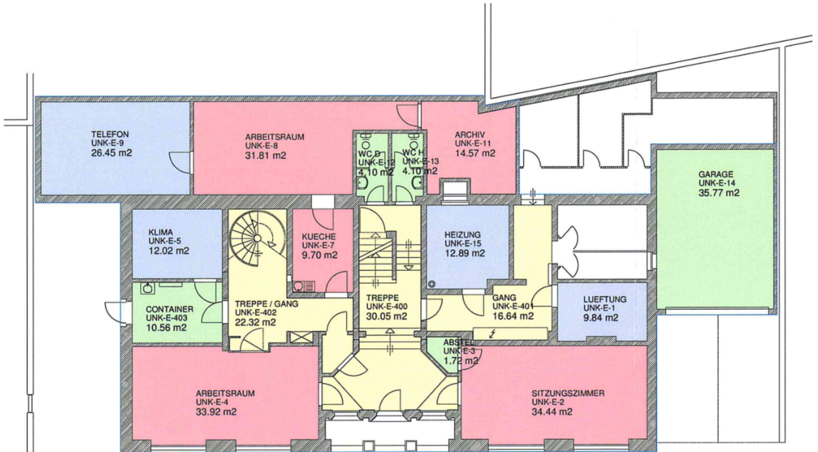
Erdgeschoss
