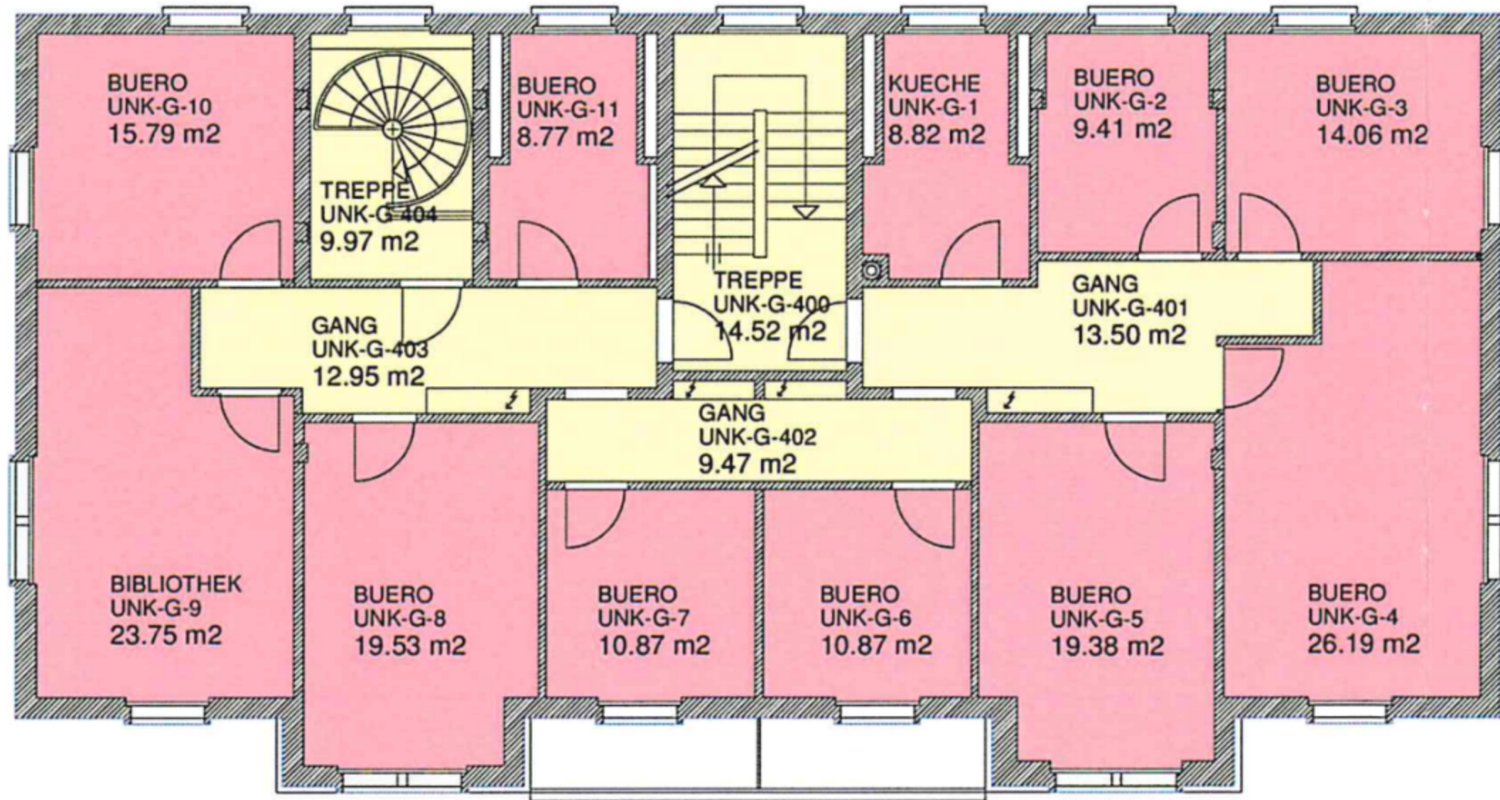
2. Obergeschoss
