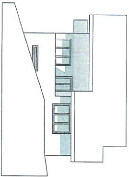
Südfassade 1:200
