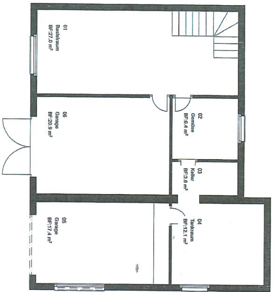
Untergeschoss 1:100
