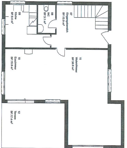
Erdgeschoss 1:100
