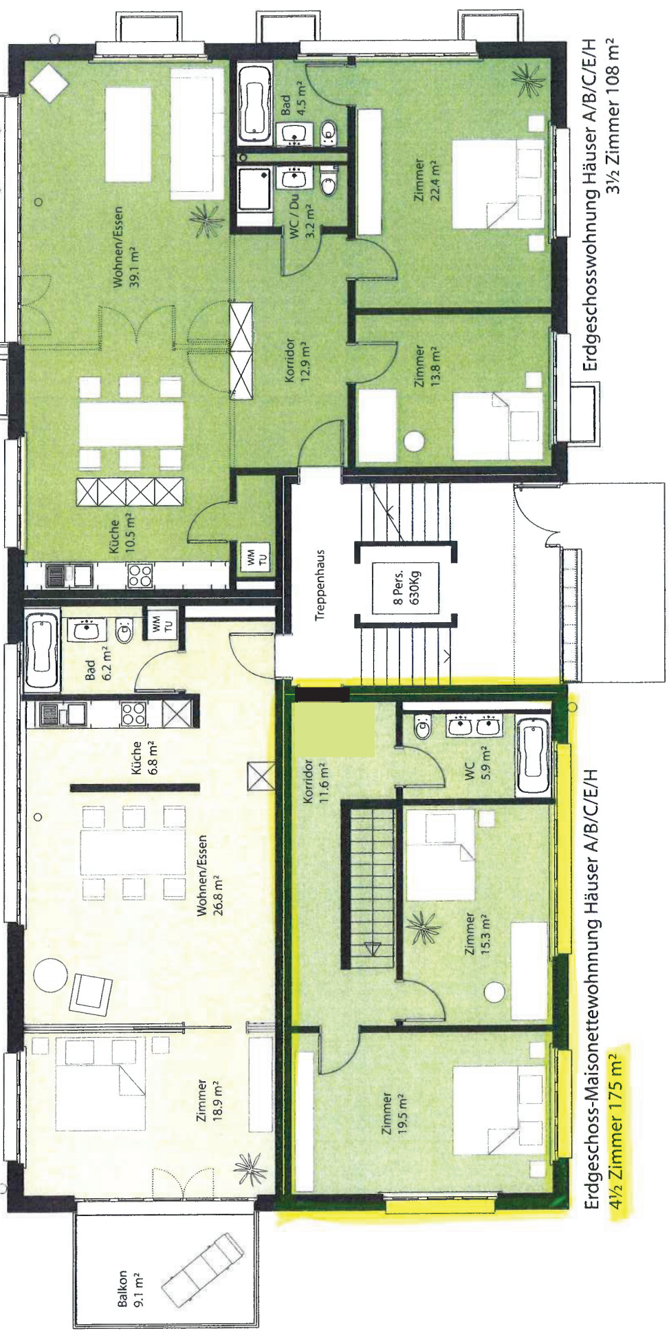
Erdgeschosswohnung Häuser A/B/C/E/H 2 Zimmer 65.2 m 2
