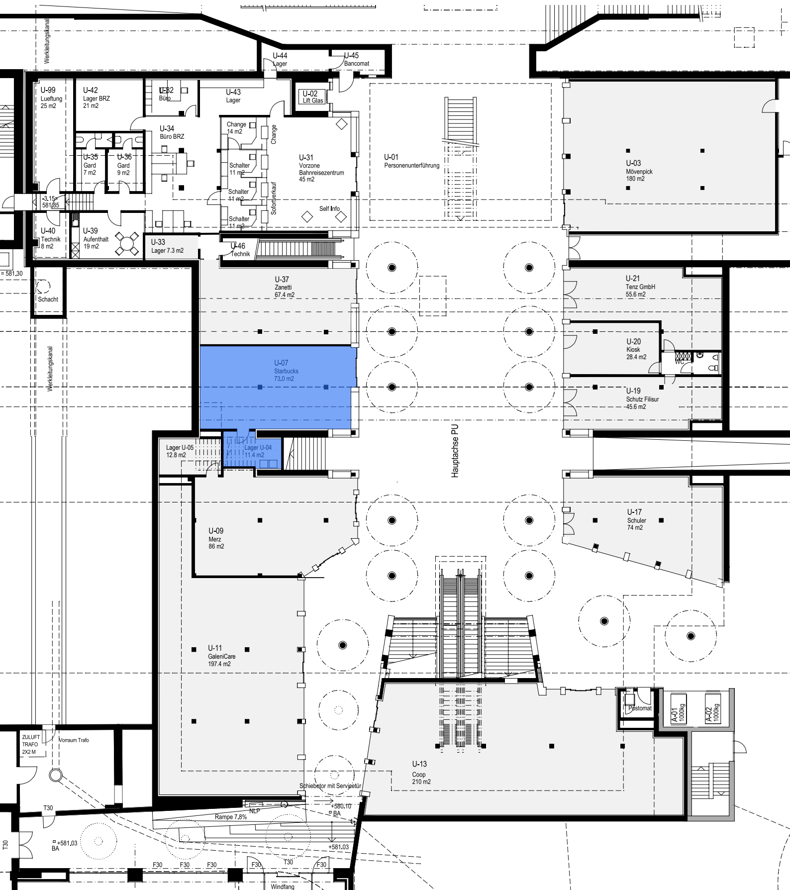
Bahnhof Chur, PU-Ladenpassage Grundriss 1. UG 1:200
