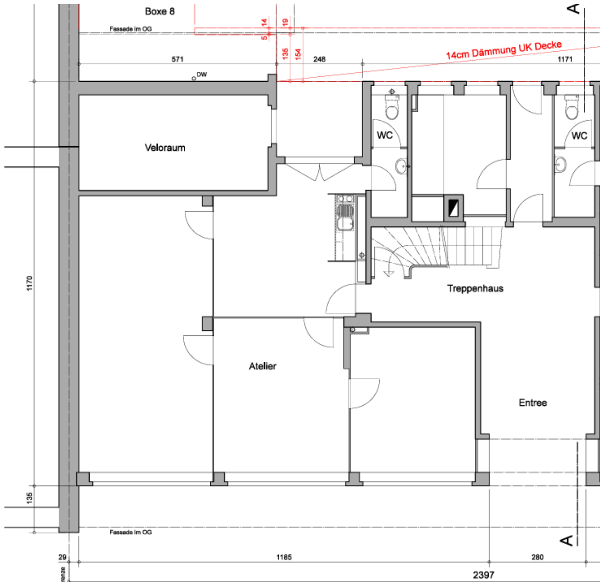
Vorderhaus Erdgeschoss
