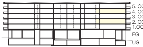
Schnitt
