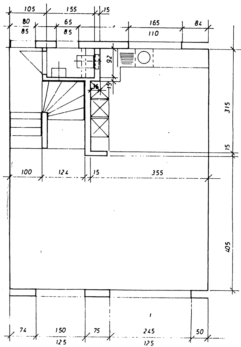
1. OBERGESCHOSS
