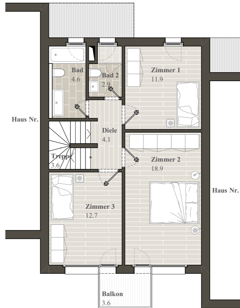
Obergeschoss 1:100
