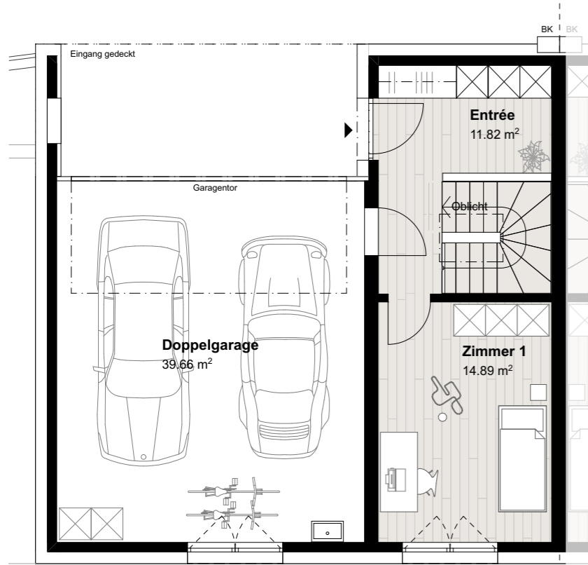
Obergeschoss 1:100
