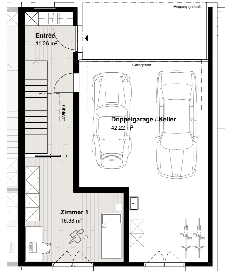
Obergeschoss 1:100
