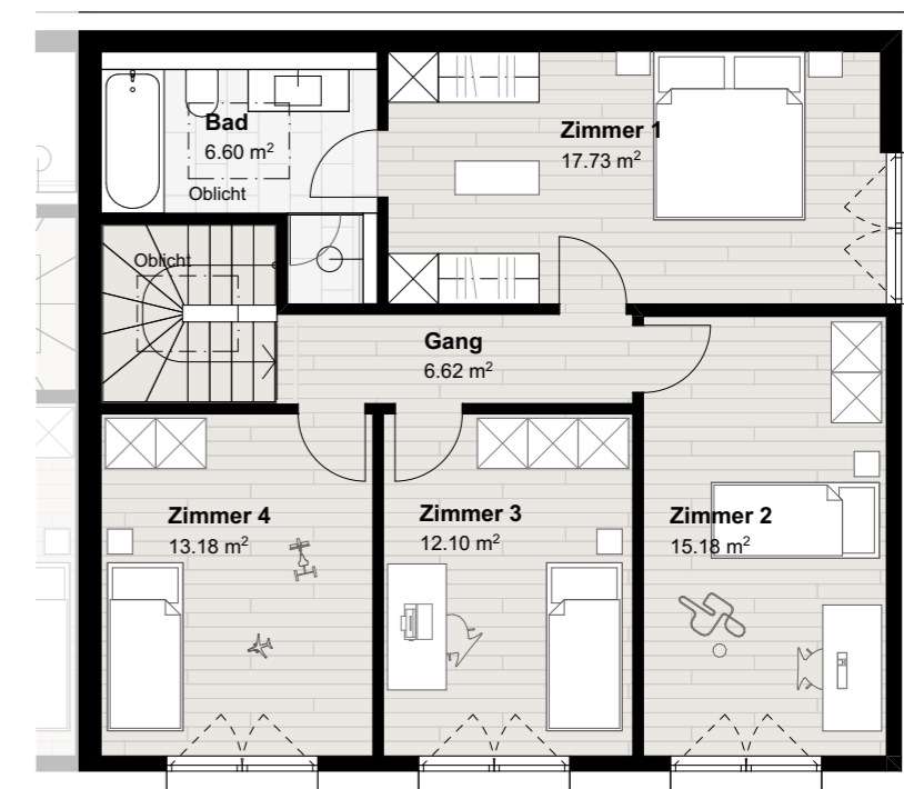
Obergeschoss 1:100
