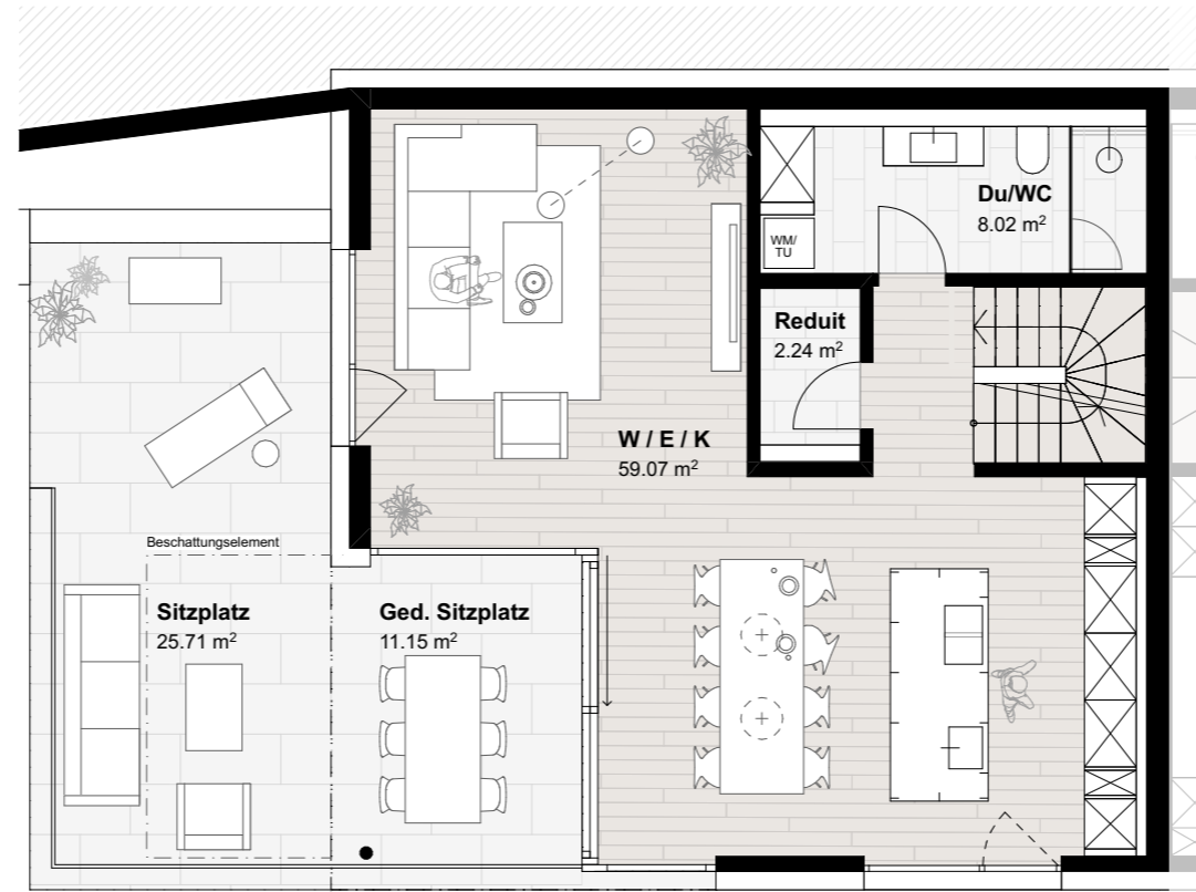
Erdgeschoss 1:100
