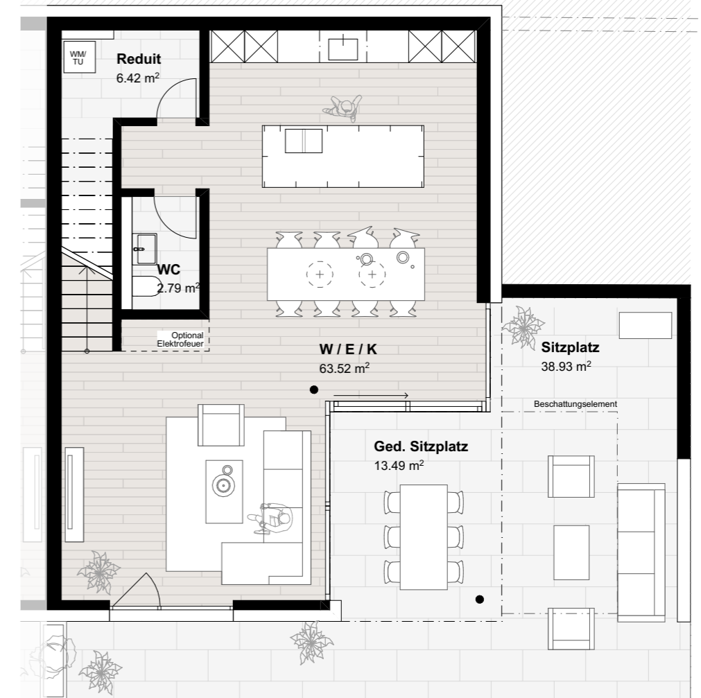
Untergeschoss 1:100
