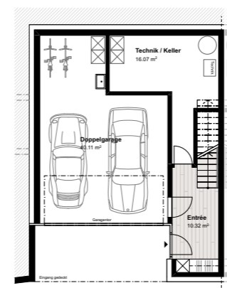
Untergeschoss 1100
