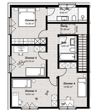
Obergeschoss 1100
