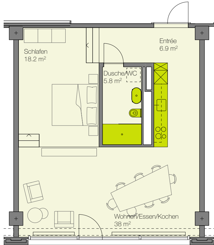
Grundriss Erdgeschoss Mst. 1:100
