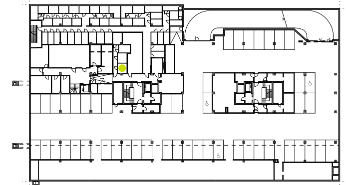
Grundriss 1. Untergeschoss Mst. 1:1000
