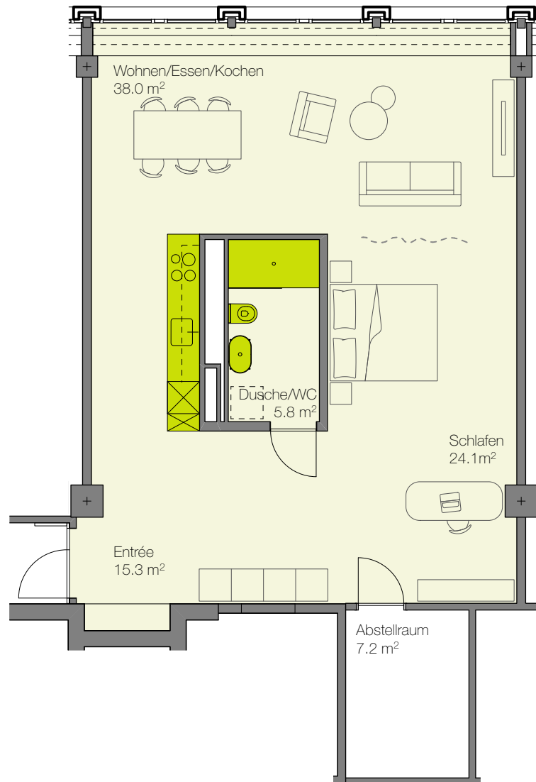
Grundriss 4. Obergeschoss Mst. 1:100
