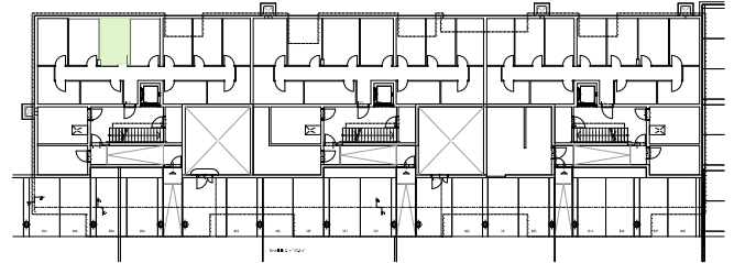
Keller UG
