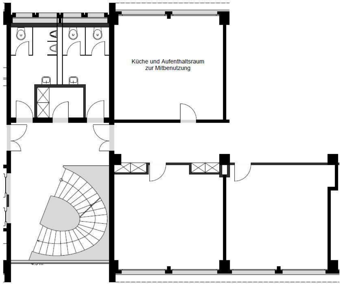
Grundrissplan
