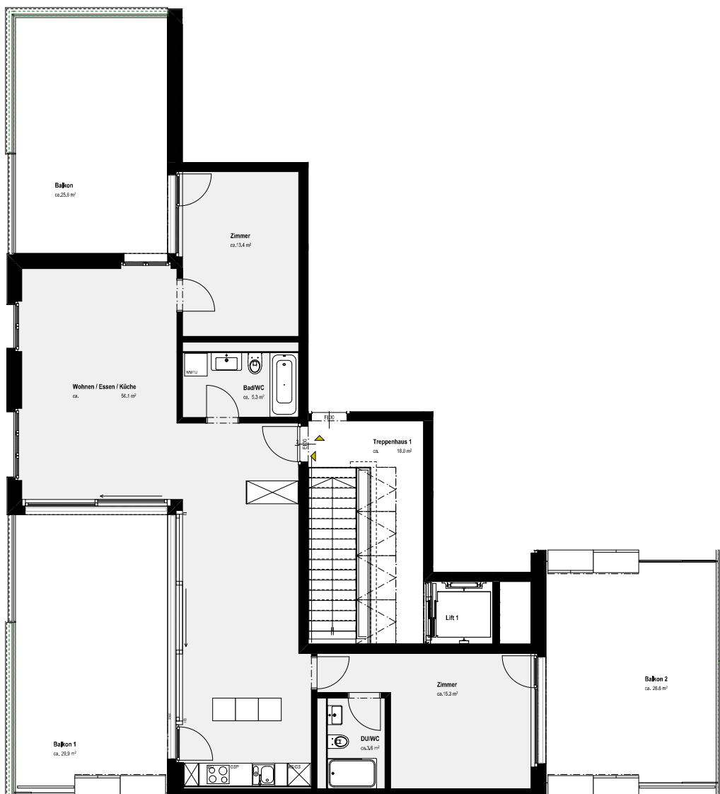
Grundriss Wohnung
