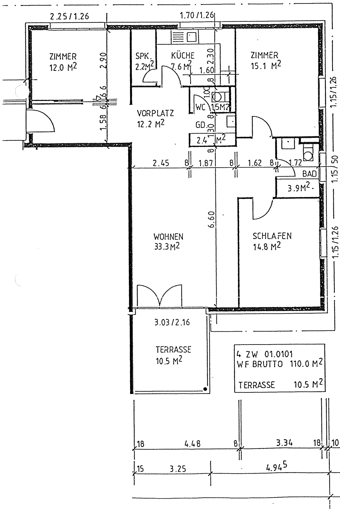
OBERGESCHOSS M. 1:100
