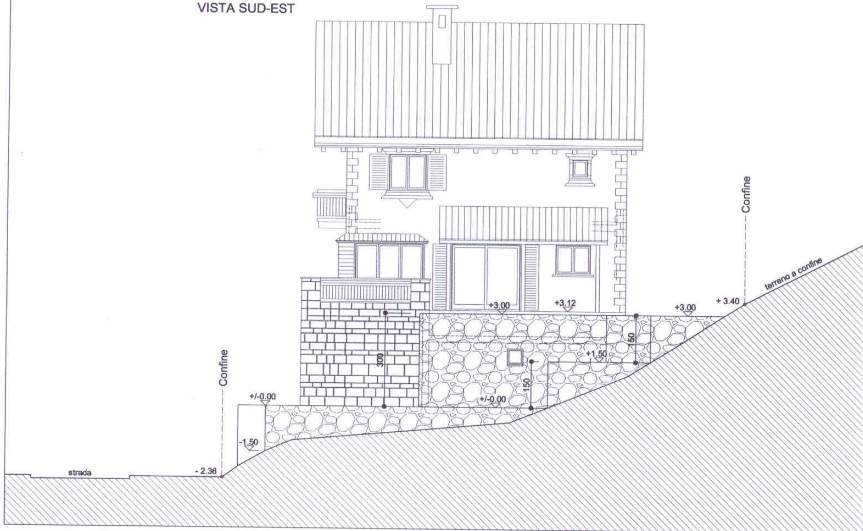
VISTA SUD-EST
